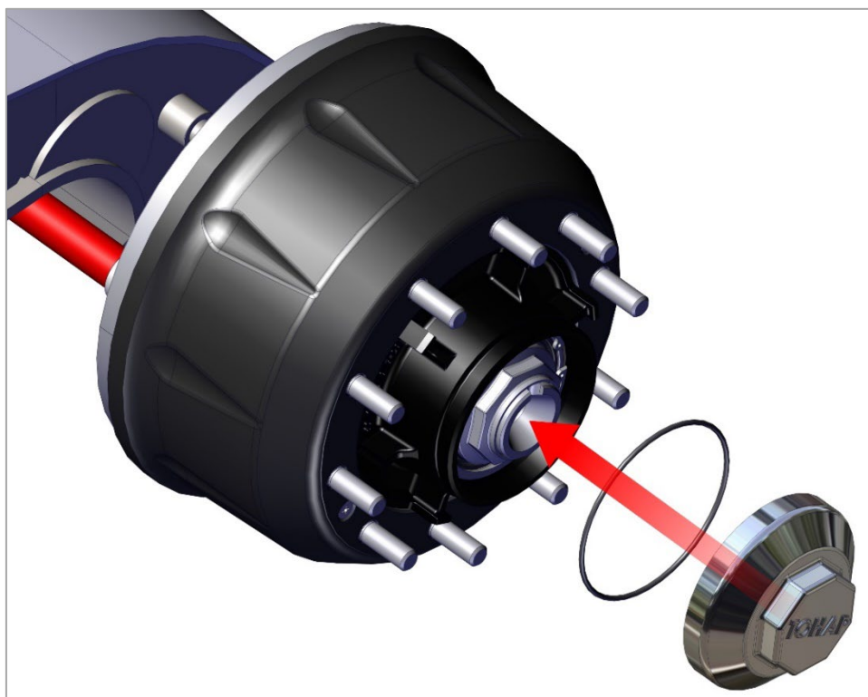
Рис. 14.2. Монтаж крышки ступицы колеса с резиновым уплотнительным кольцом.
