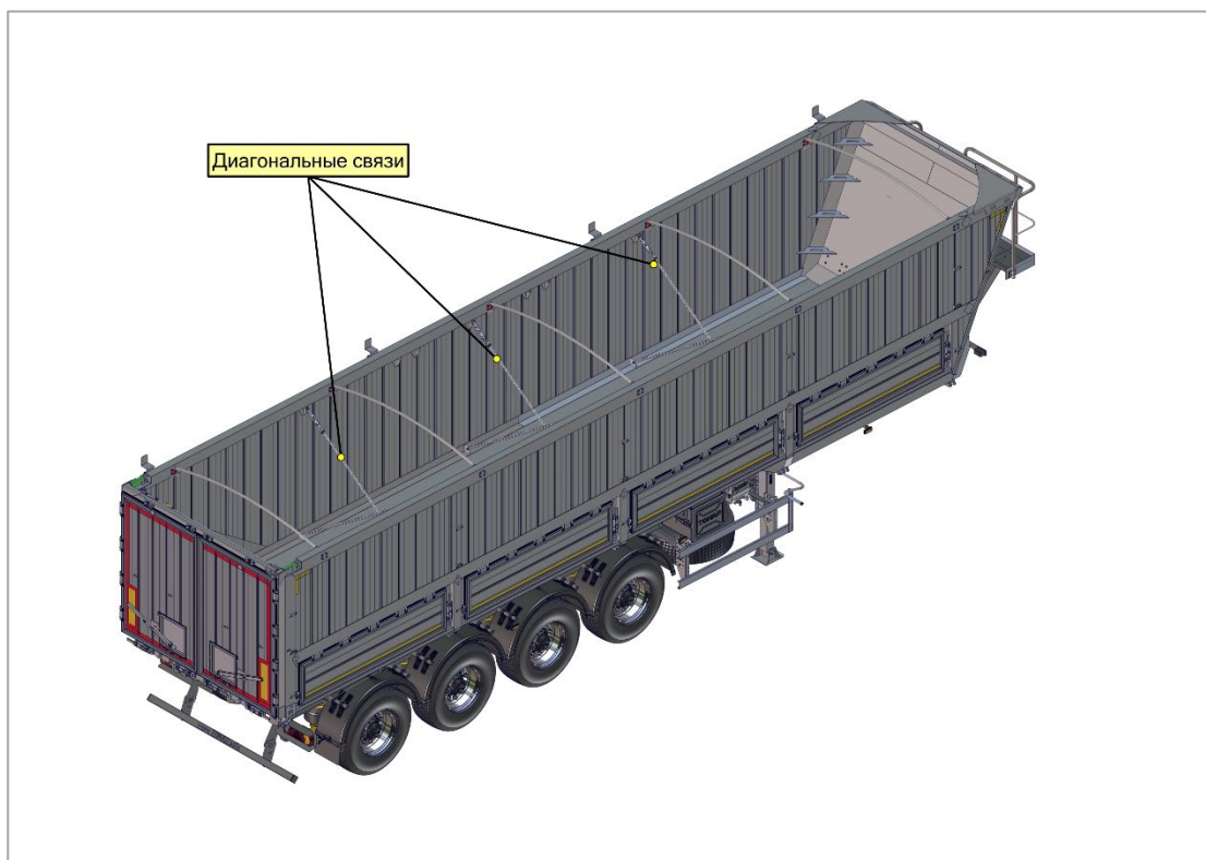
Рис. 1. Диагональные связи
