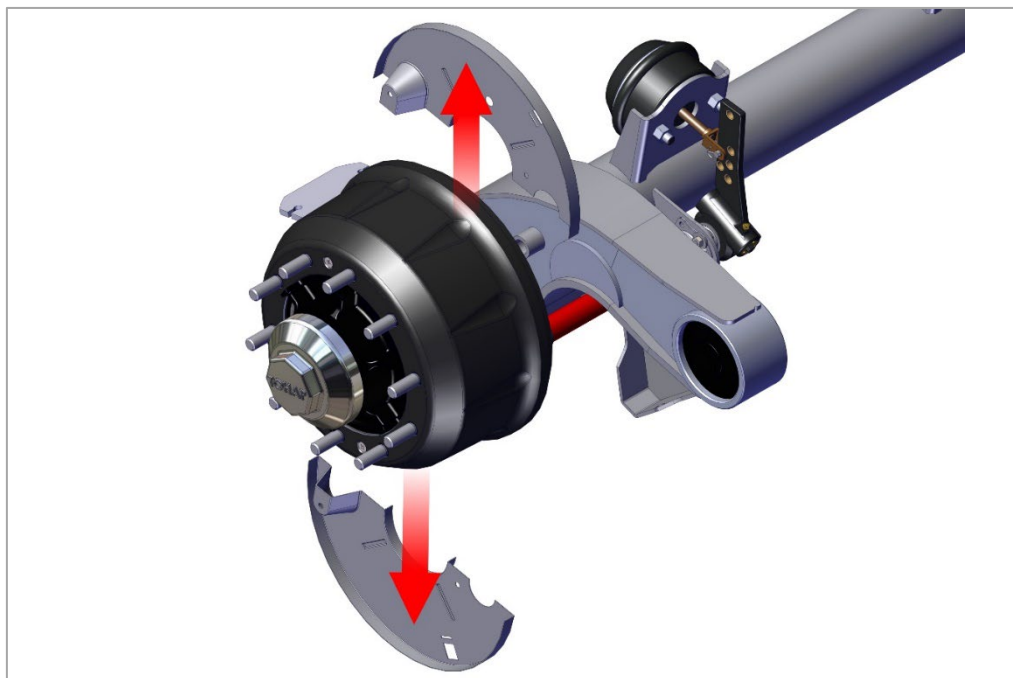
Рис. 18. Снятие грязезащитных щитков.
