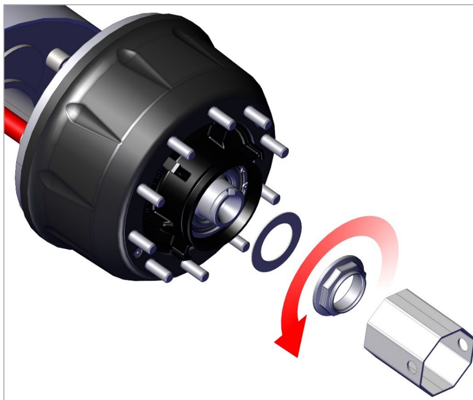
Рис. 12. Снятие гайки подшипников.
