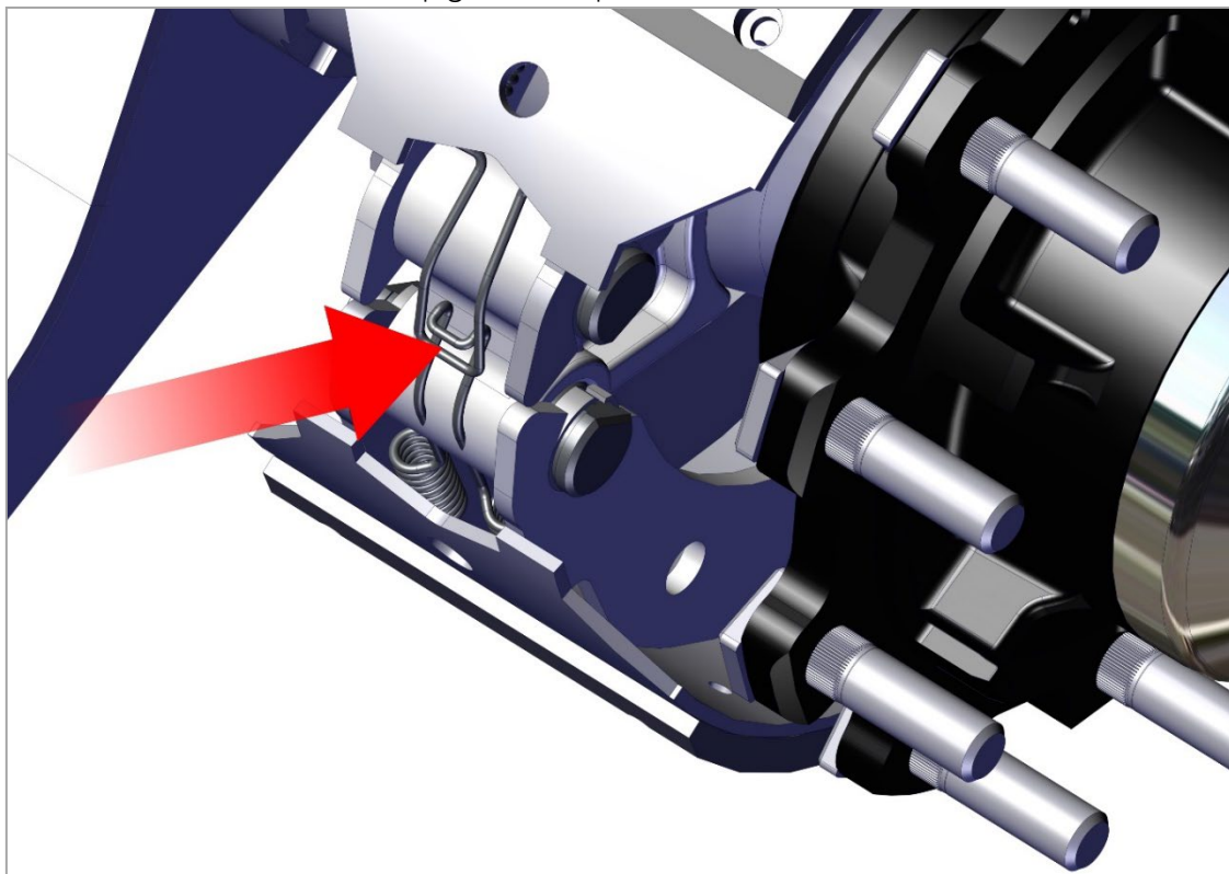
Рис. 20. Зажим пружины.
