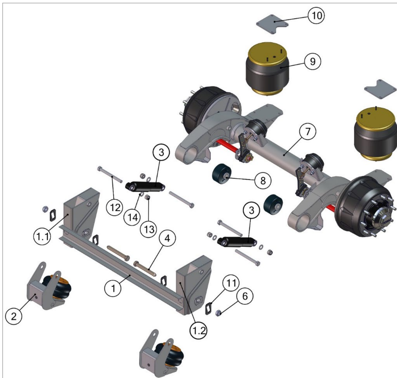
Рис. 5. Взрыв-схема рычажной подвески с барабанными тормозами.
