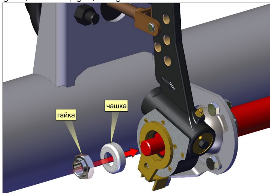
Рис. 23.3. Закрепить регулятор.
