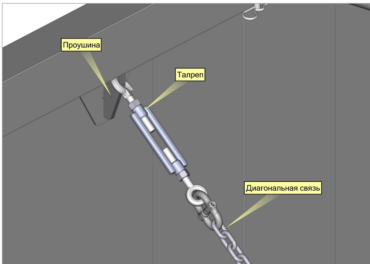
Рис. 2. Крепление диагональных связей к кузову
