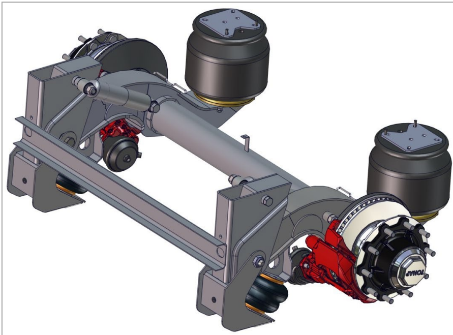
Рис. 4. Рычажная подвеска с дисковыми тормозами.
