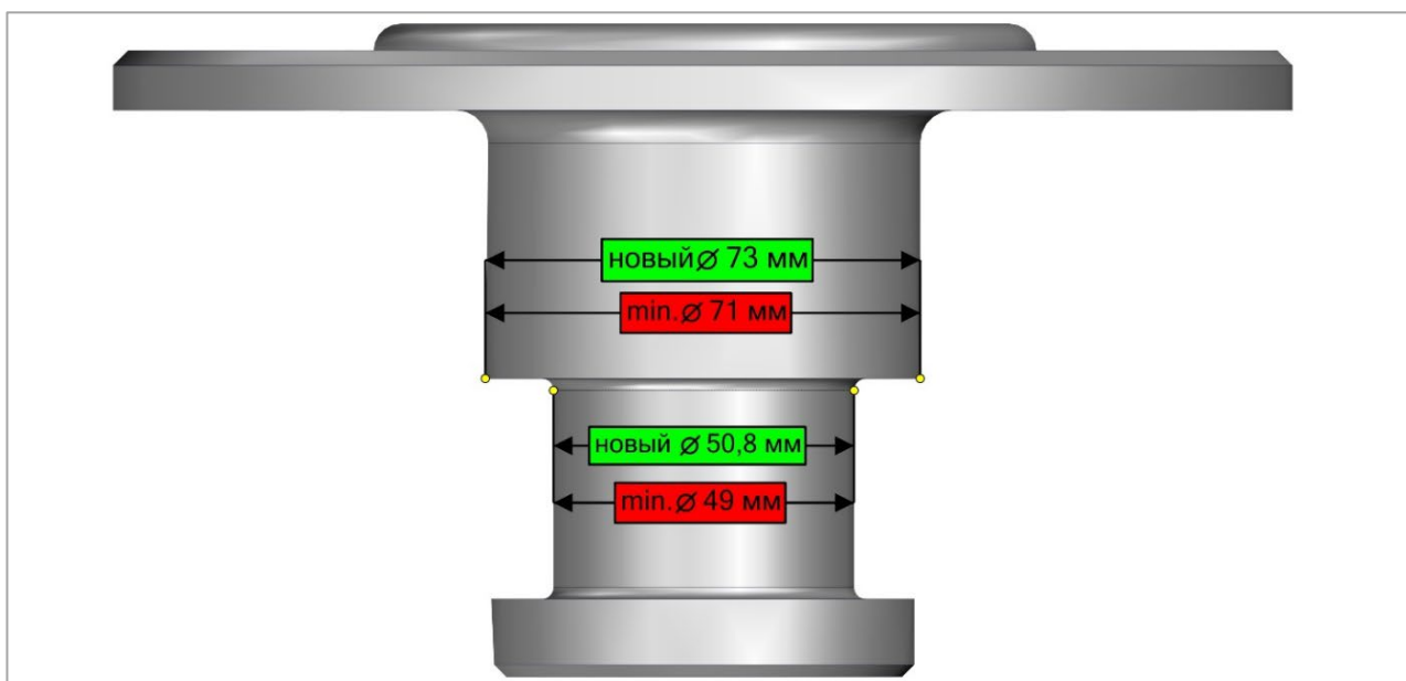
Рис. 33. Шкворень
