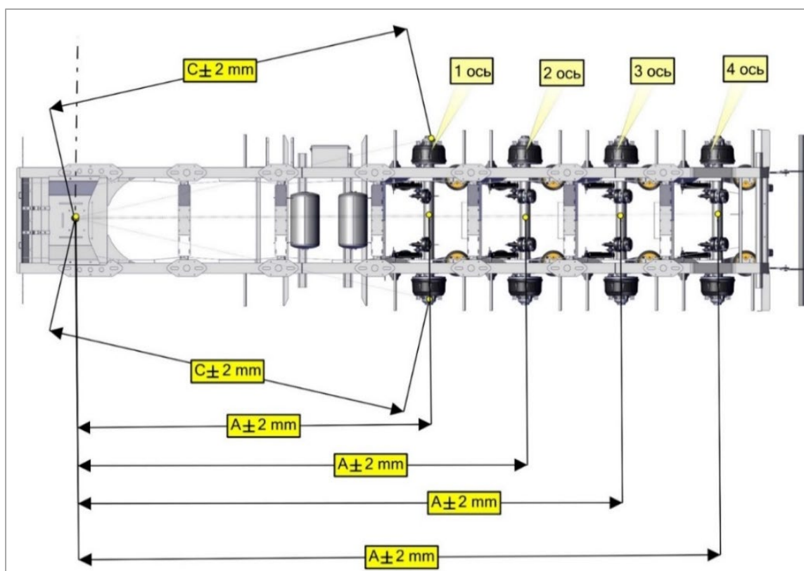
Рис. 27.2. Регулировка осей.
