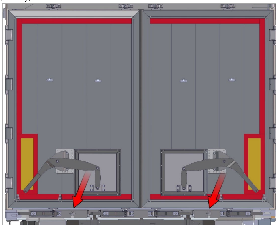
Рис. 37.1. Положение рым-гаек
