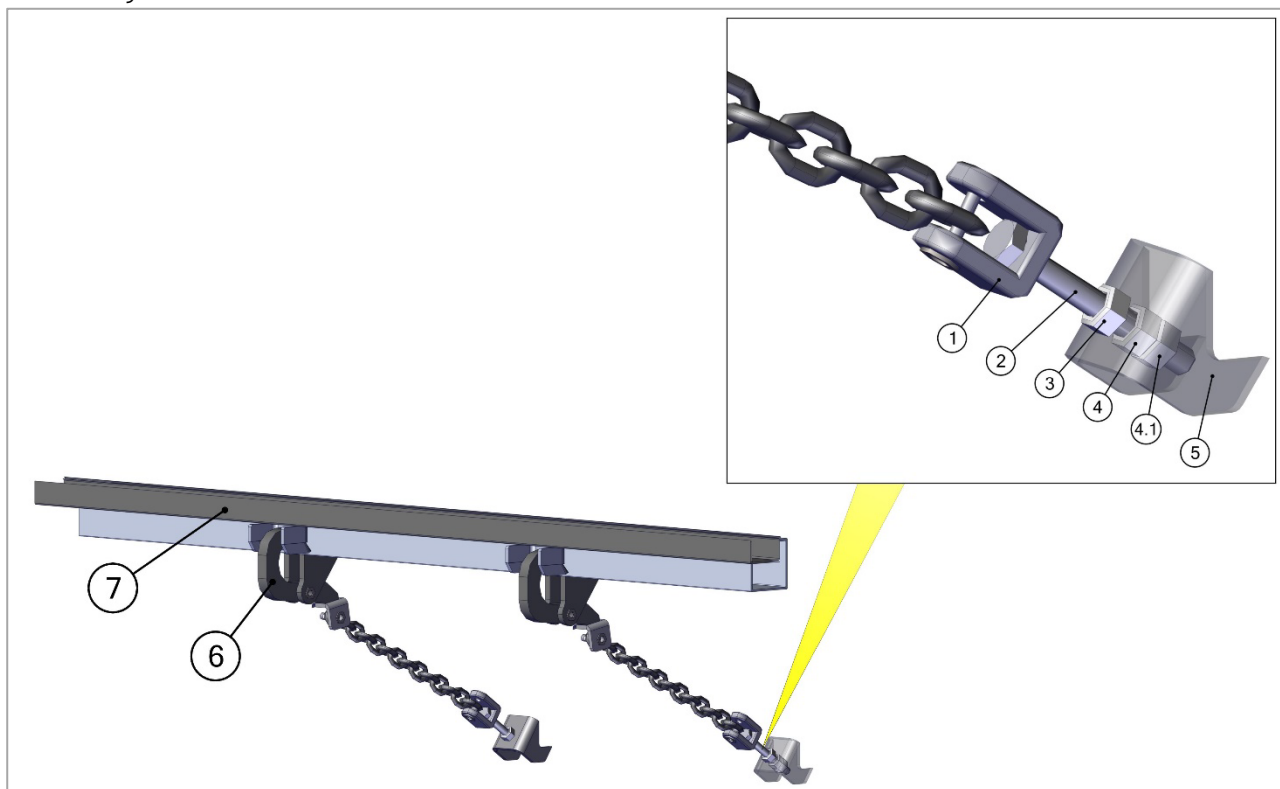
Рис. 36. Механизм запираие борта
