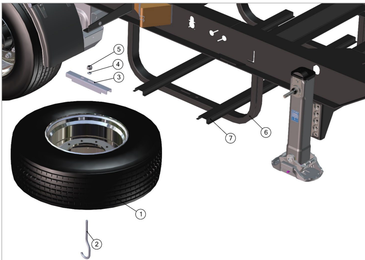
Рис. 35. Запасное колесо
