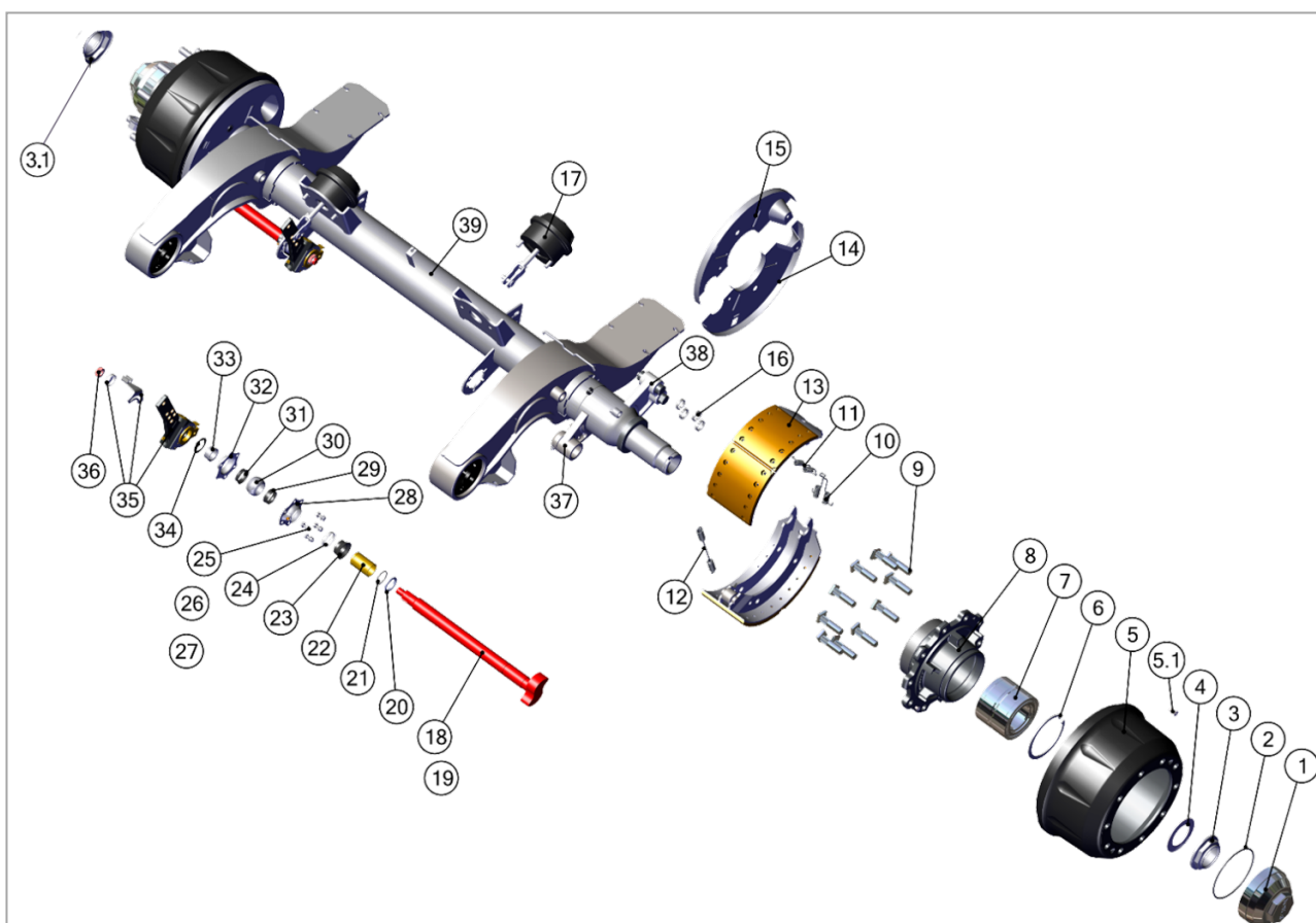
Рис. 8. Взрыв-схема оси полуприцепа с барабанными тормозами.
