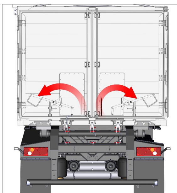
Рис. 39.1; 39.2; 39.3. Порядок открытия
