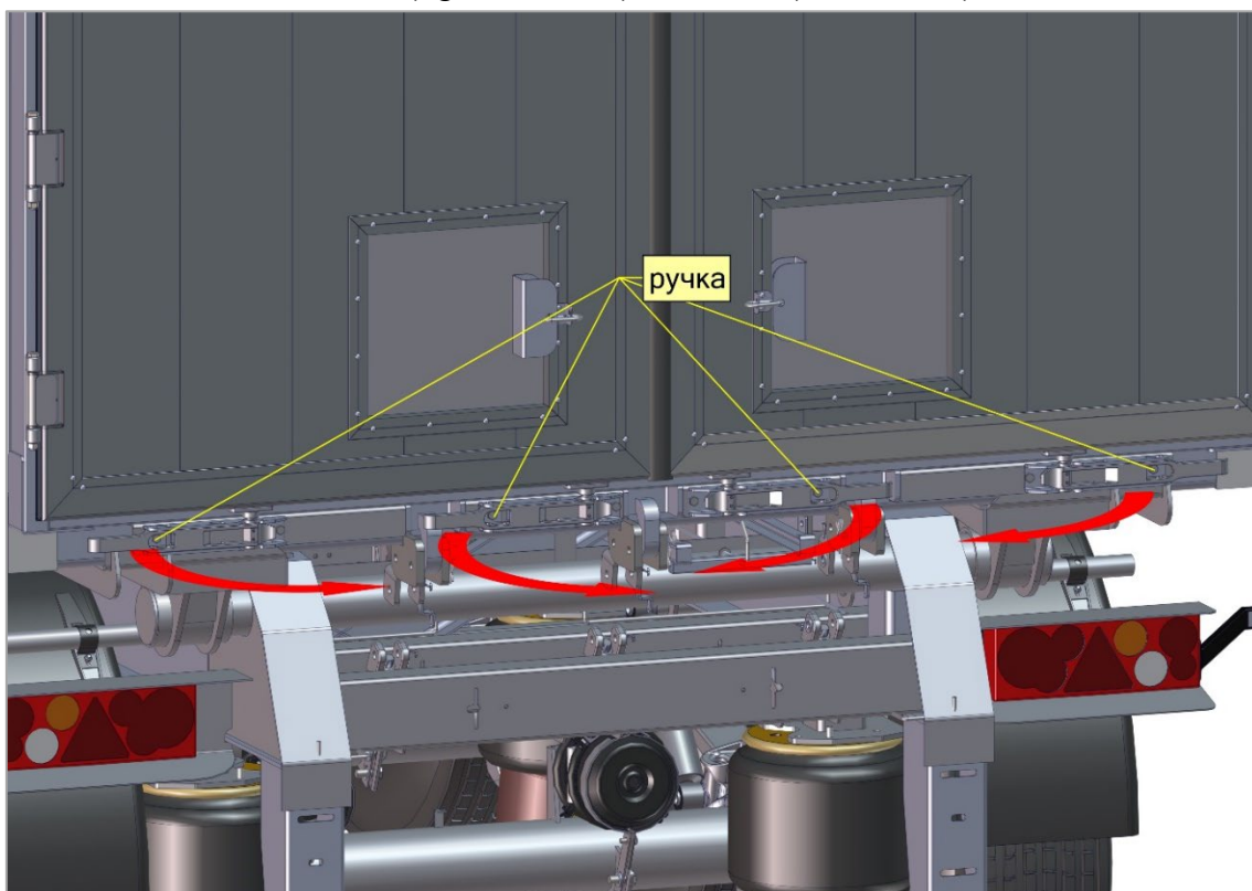
Рис. 41.2. Открытие дверей с помощью ручек
