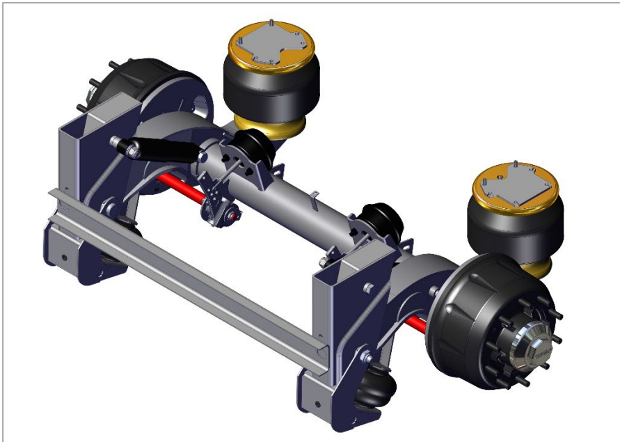
Рис. 3. Рычажная подвеска с барабанными тормозами.
