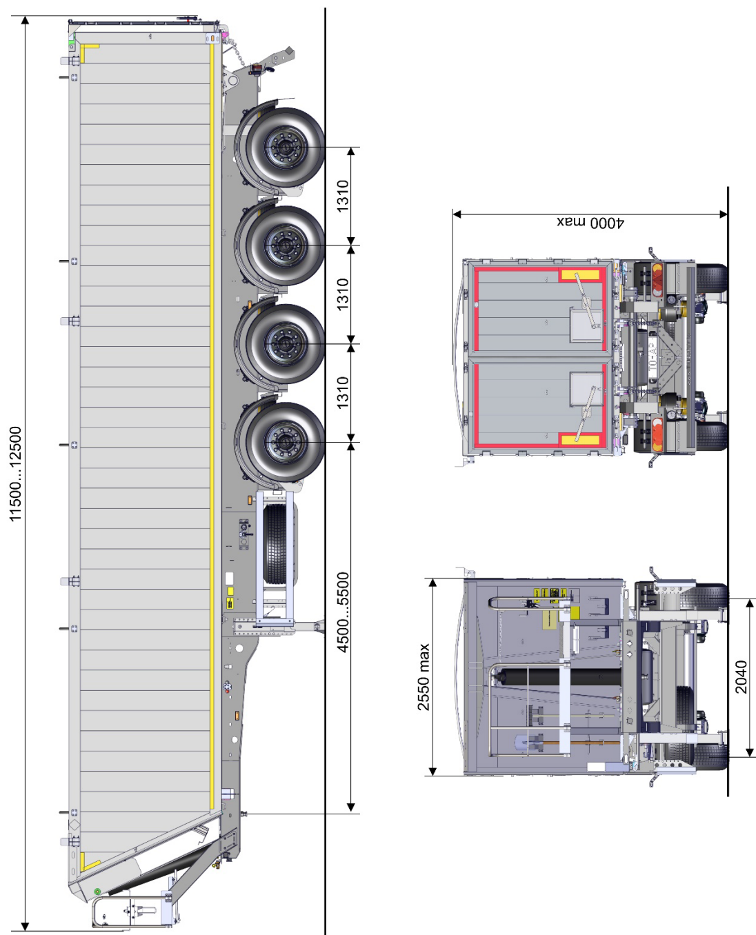
Рис.44. Габаритный чертёж 95991
