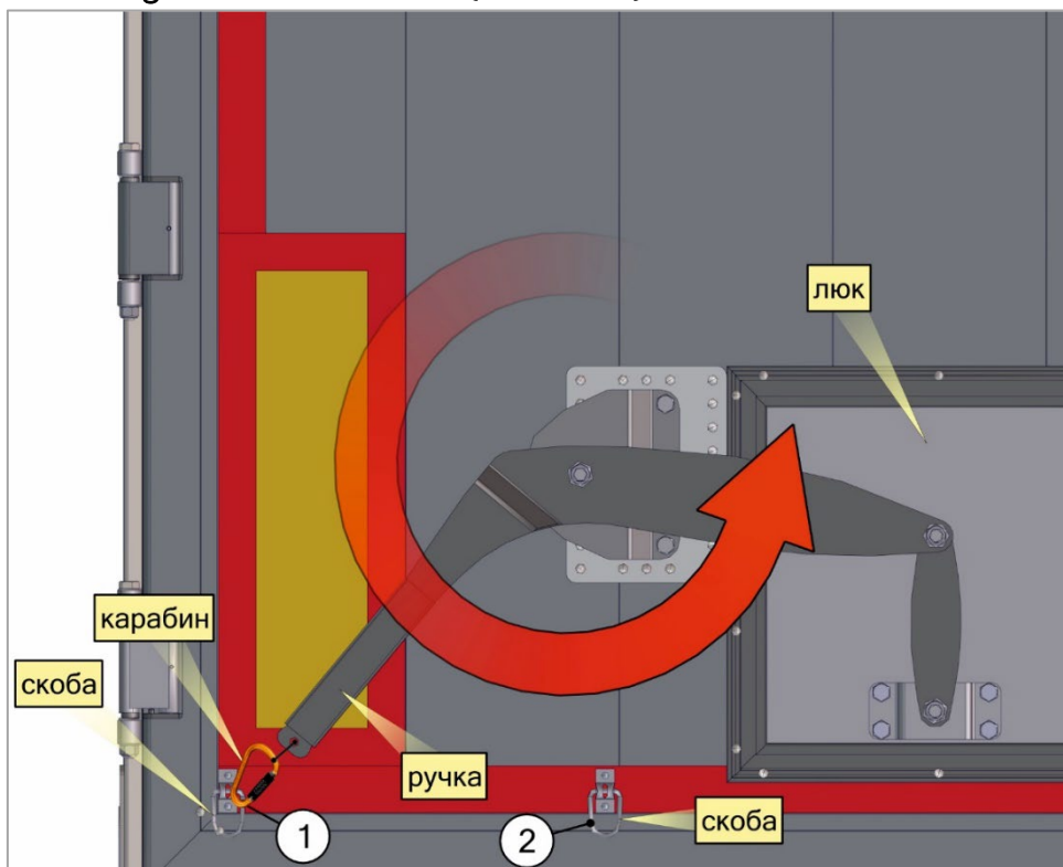
Рис. 40.1 Фиксация люков
