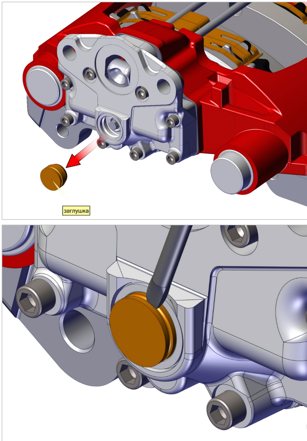
Рис. 28; 28.1. Удаление заглушки.
