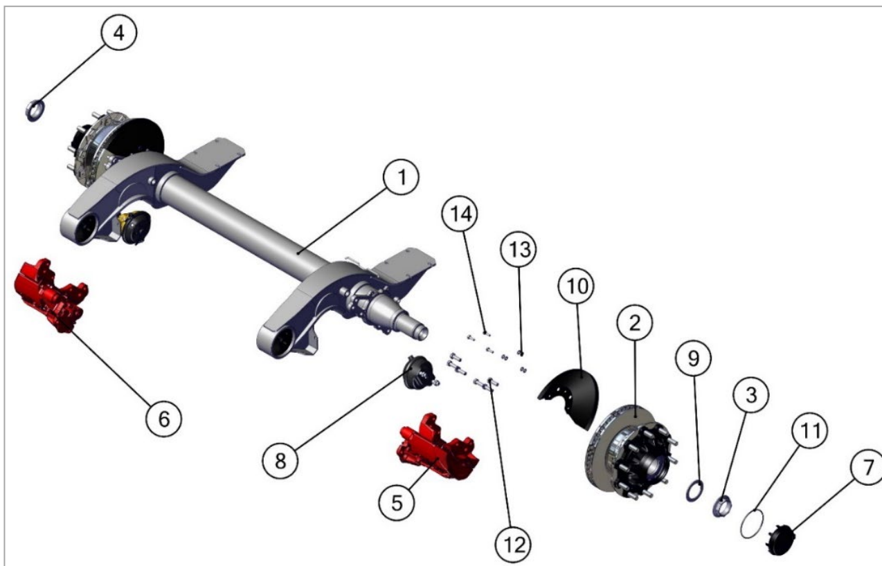
Рис. 25. Взрыв-схема оси с дисковыми тормозами.
