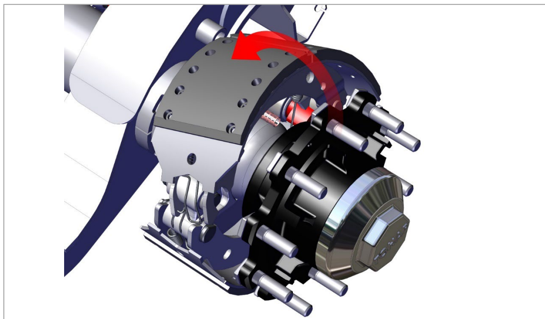
Рис. 21. Снятие тормозной колодки.
