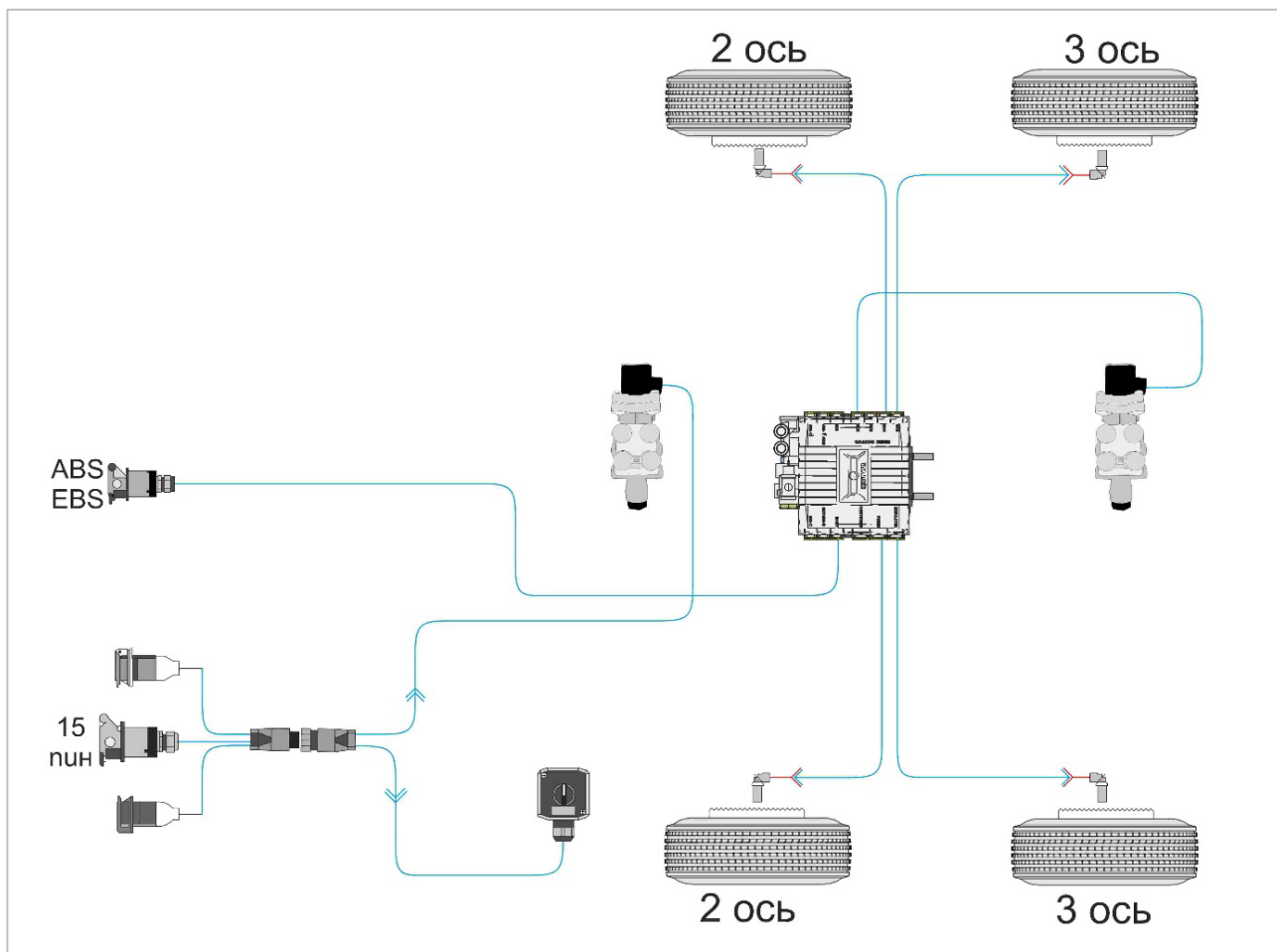
Рис. 29.3. Электрическая схема (для моделей с автоматическим управлением подъёмными осями)
