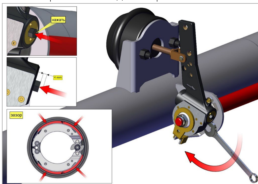
Рис. 23.7. Фиксатор.
