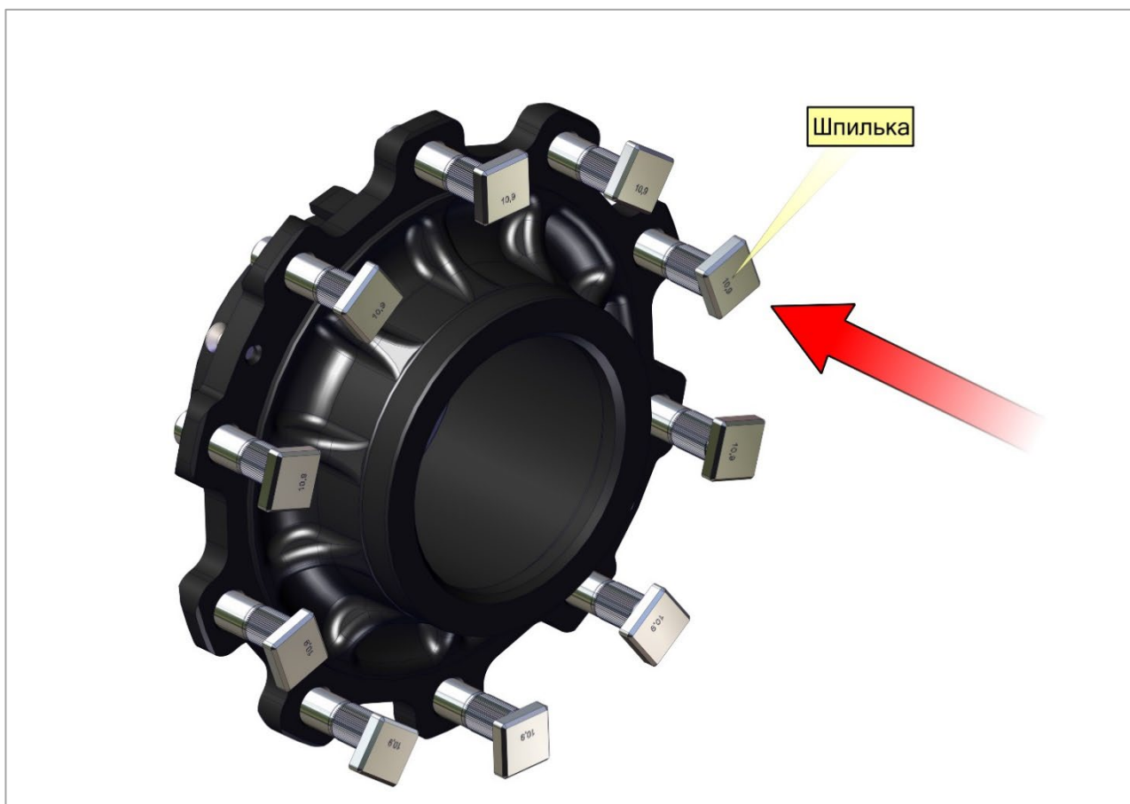
Рис. 15. Установка шпилек.
