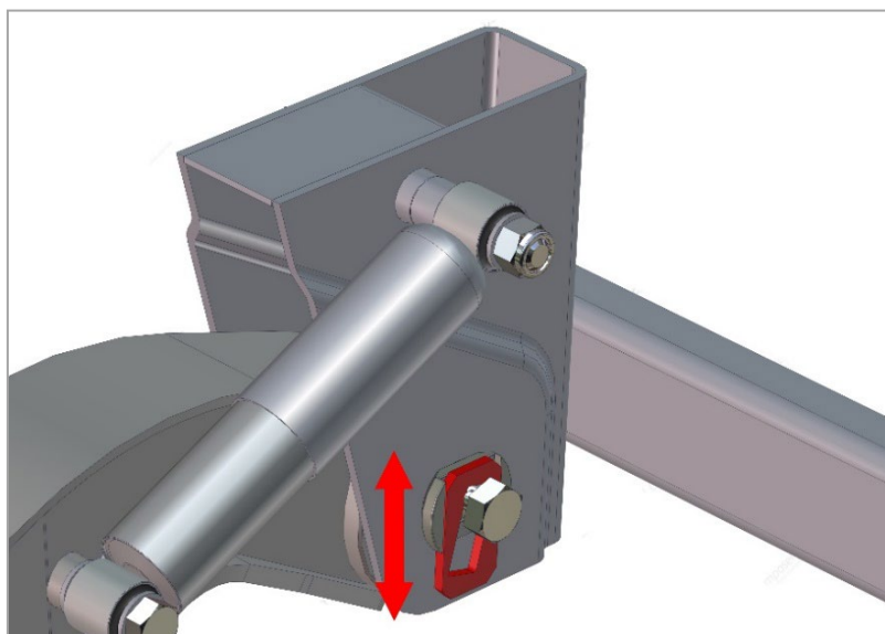
Рис. 27.1. Регулировочные пластины.
