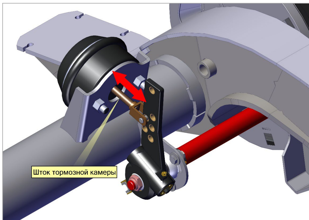
Рис. 22. Шток тормозных камер.
