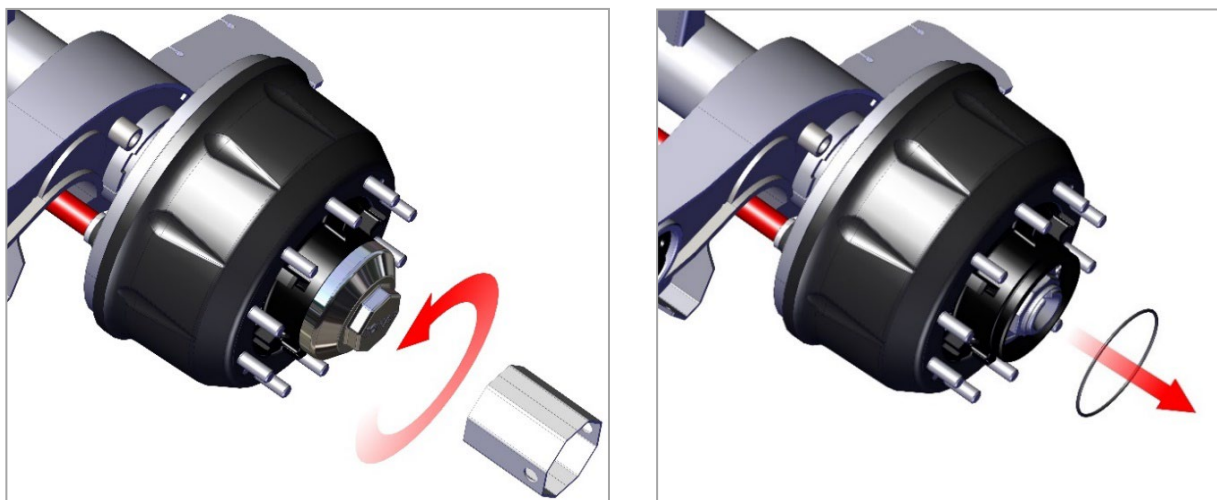
Рис. 11. Снятие крышки ступицы.
