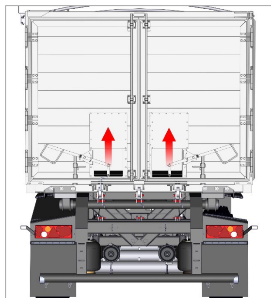
Рис. 39.1; 39.2; 39.3. Порядок открытия
