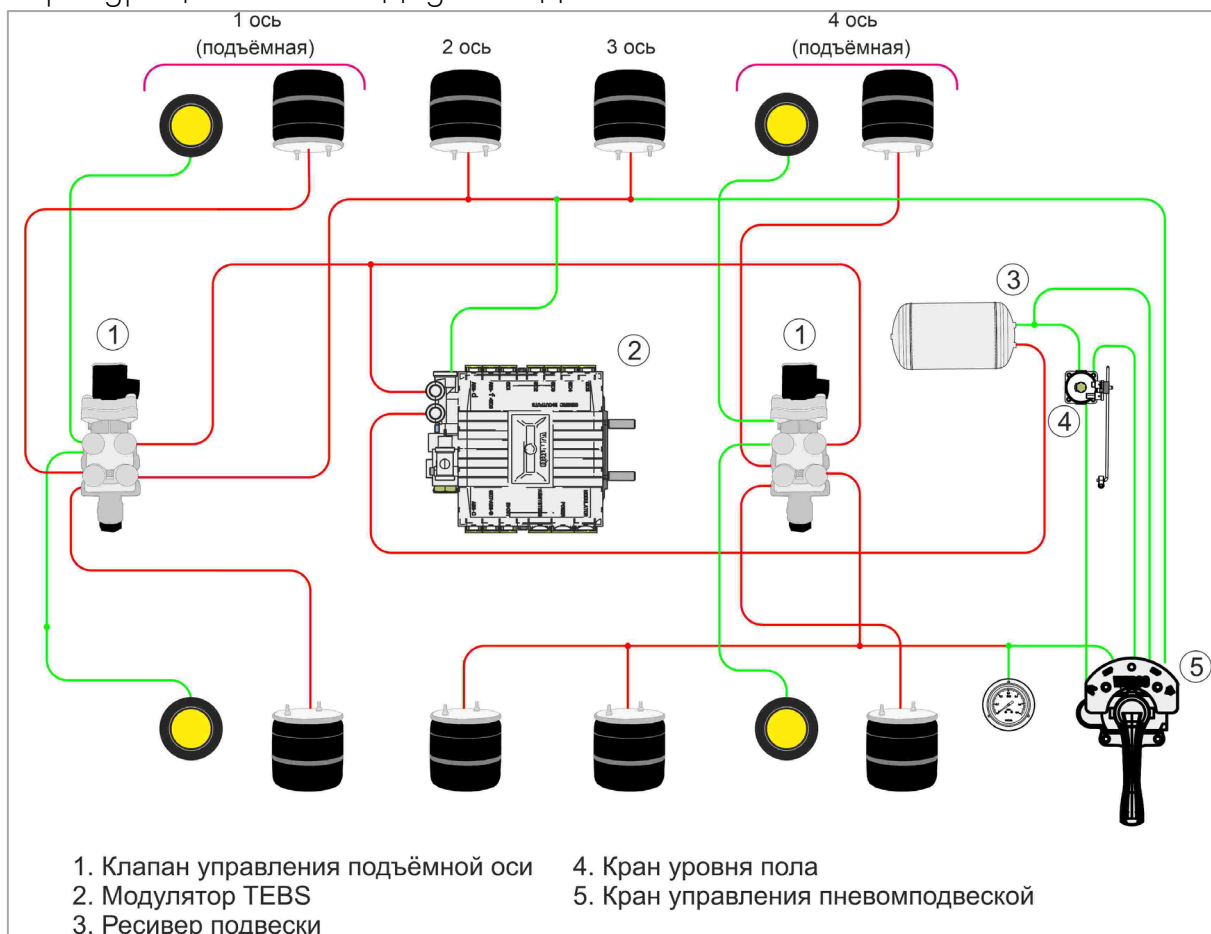
Рис. 29. Контур пневмоподвески
