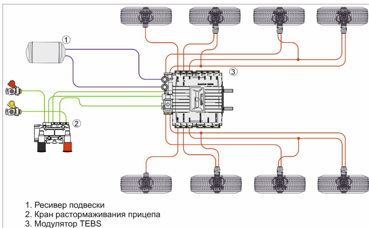
Рис. 29.1. Тормозной контур
