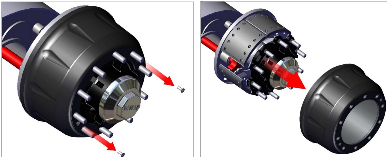
Рис. 12.2. и рис. 12.3. Снятие барабана.
