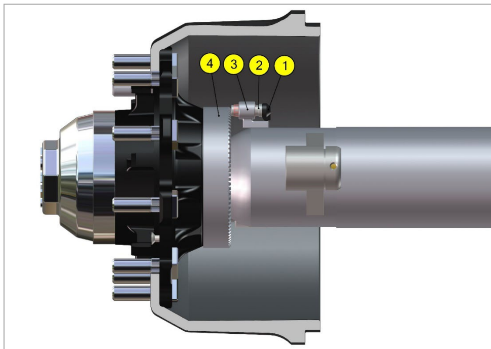
Рис. 9. Датчики ABS
