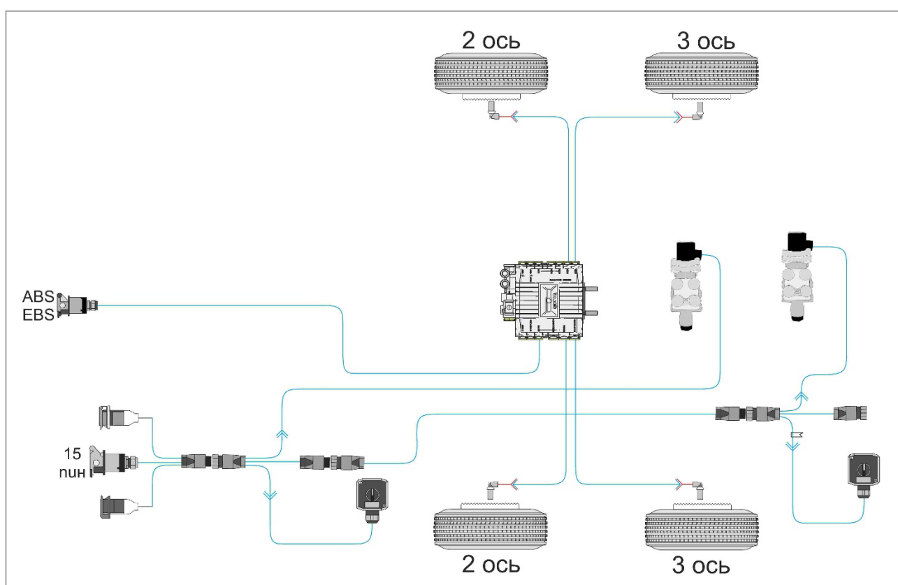
Рис. 29.2. Электрическая схема (для моделей с ручным управлением подъёмными осями)
