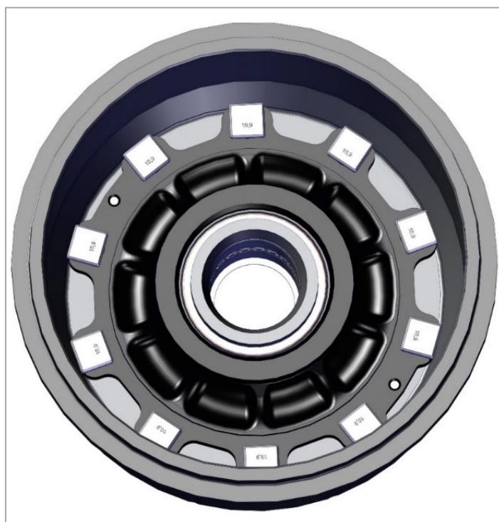
Рис. 12.1. Снятие сборочного узла ступицы и барабана.
