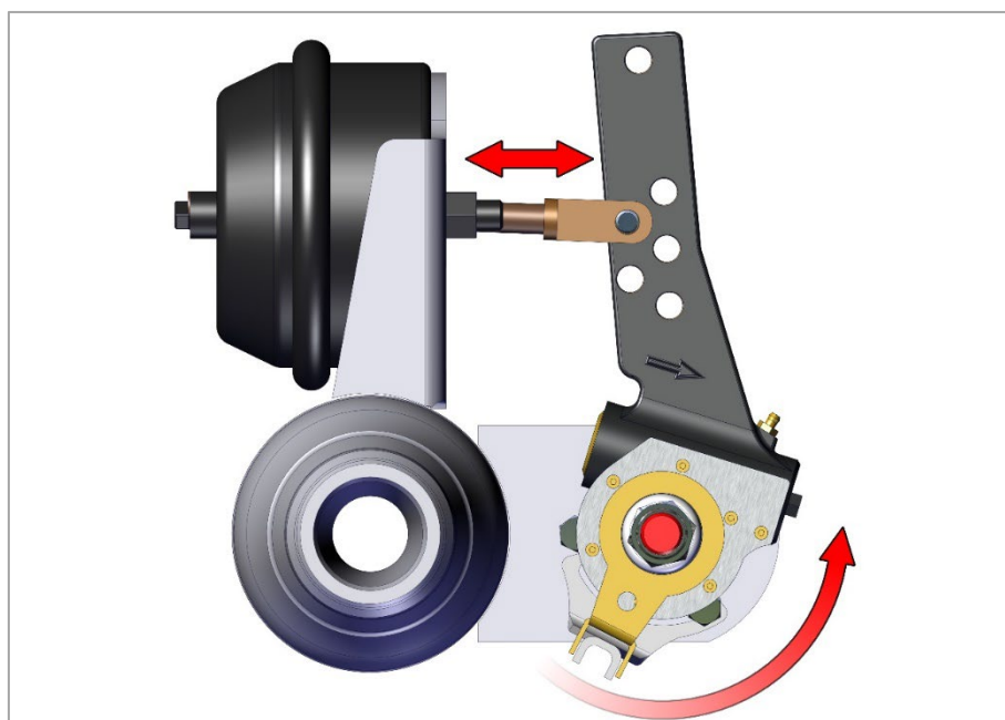
Рис. 23.4. Закрепить регулятор.
