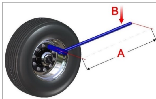
Рис. 30.1. Затяжка гаек
