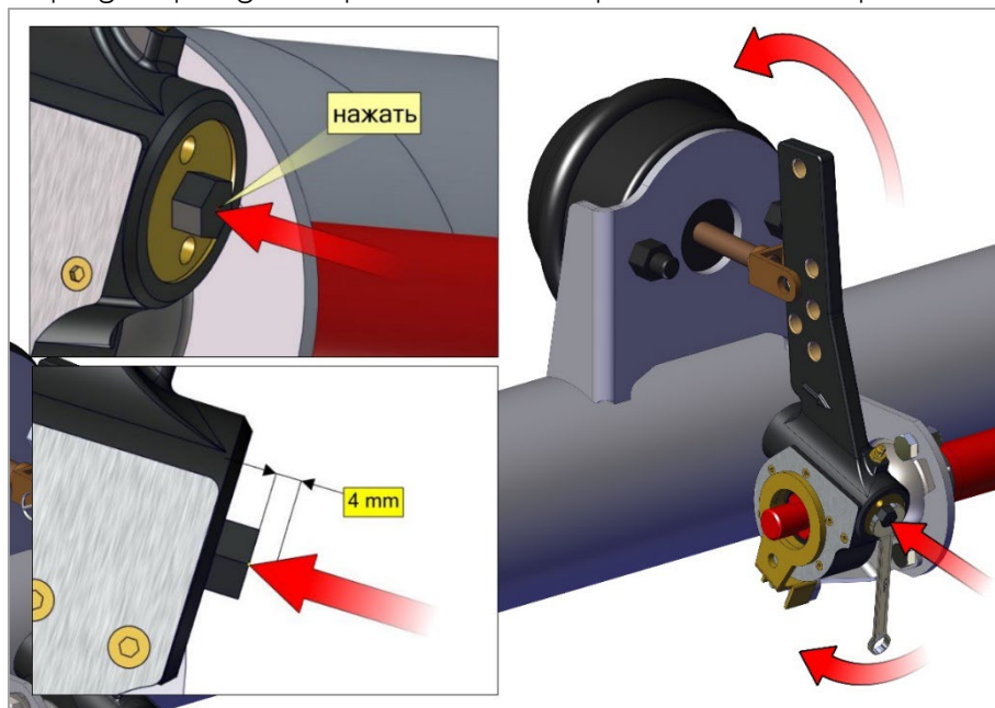
Рис. 23.1. Фиксатор.
