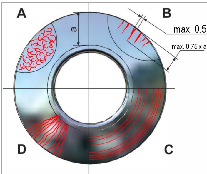
Рис. 29. Состояние рабочих поверхностей.
