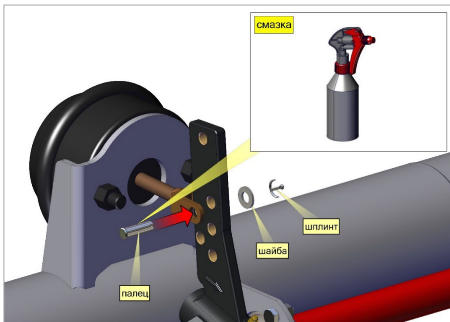
Рис. 23.2. Установка регулятора.
