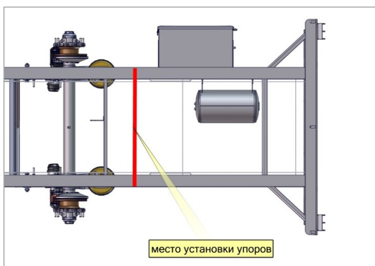
Рис. 26.1. Место установки упоров.
