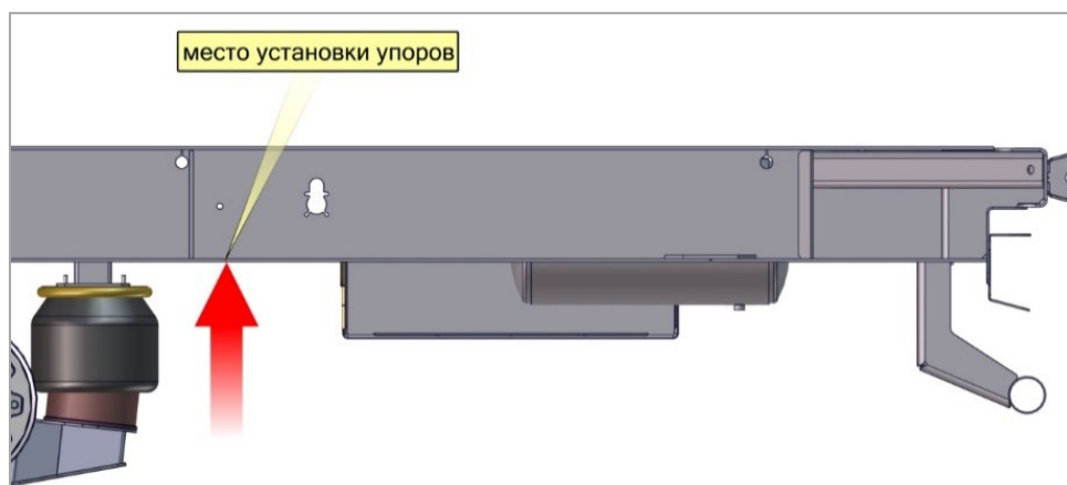
Рис. 26. Место установки упоров.
