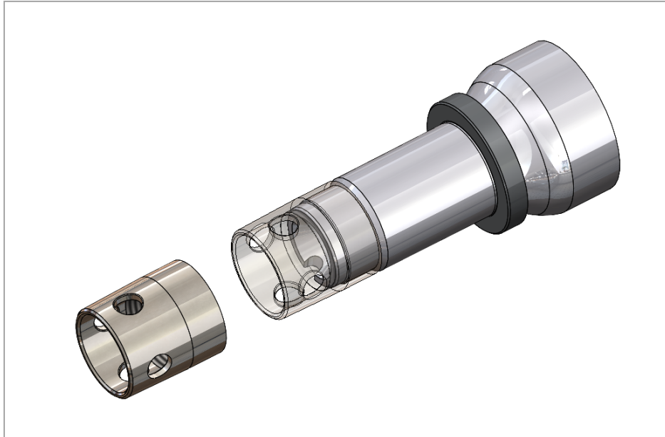
Рис. 10. Установка муфты защиты на резьбу цапфы.
