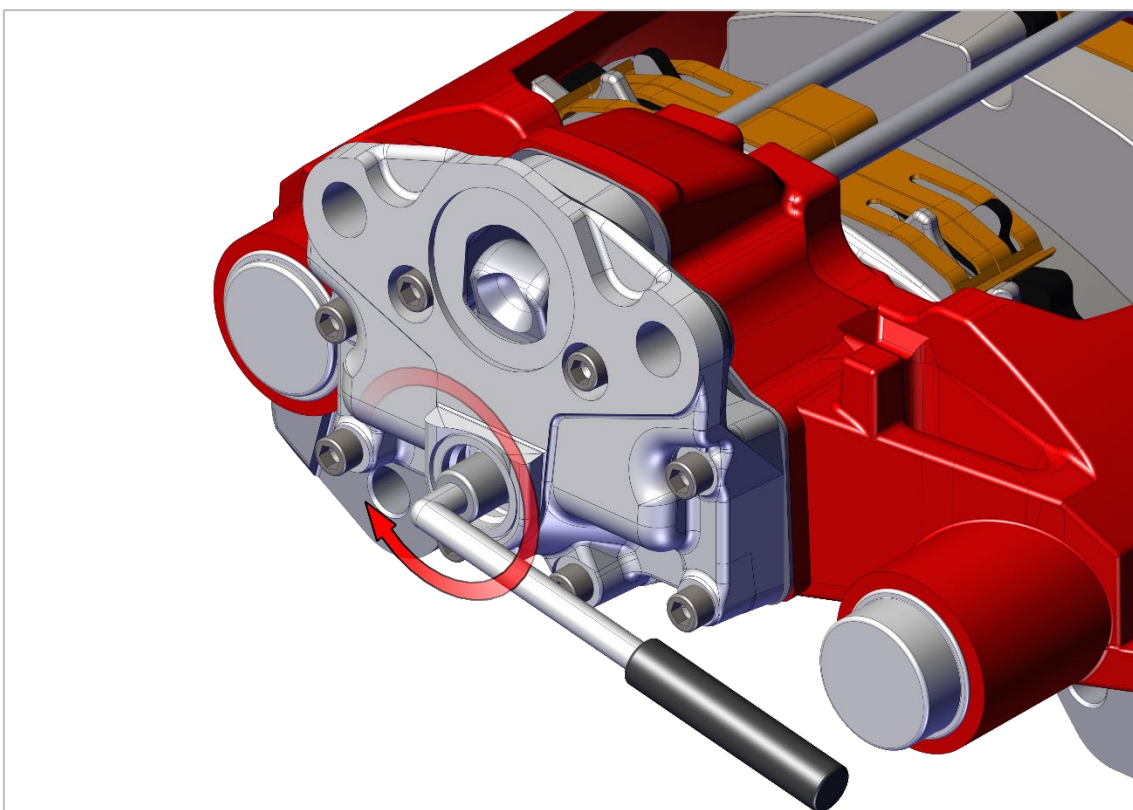
Рис. 28.2; 28.3. Проверка исправности тормозного механизма.
