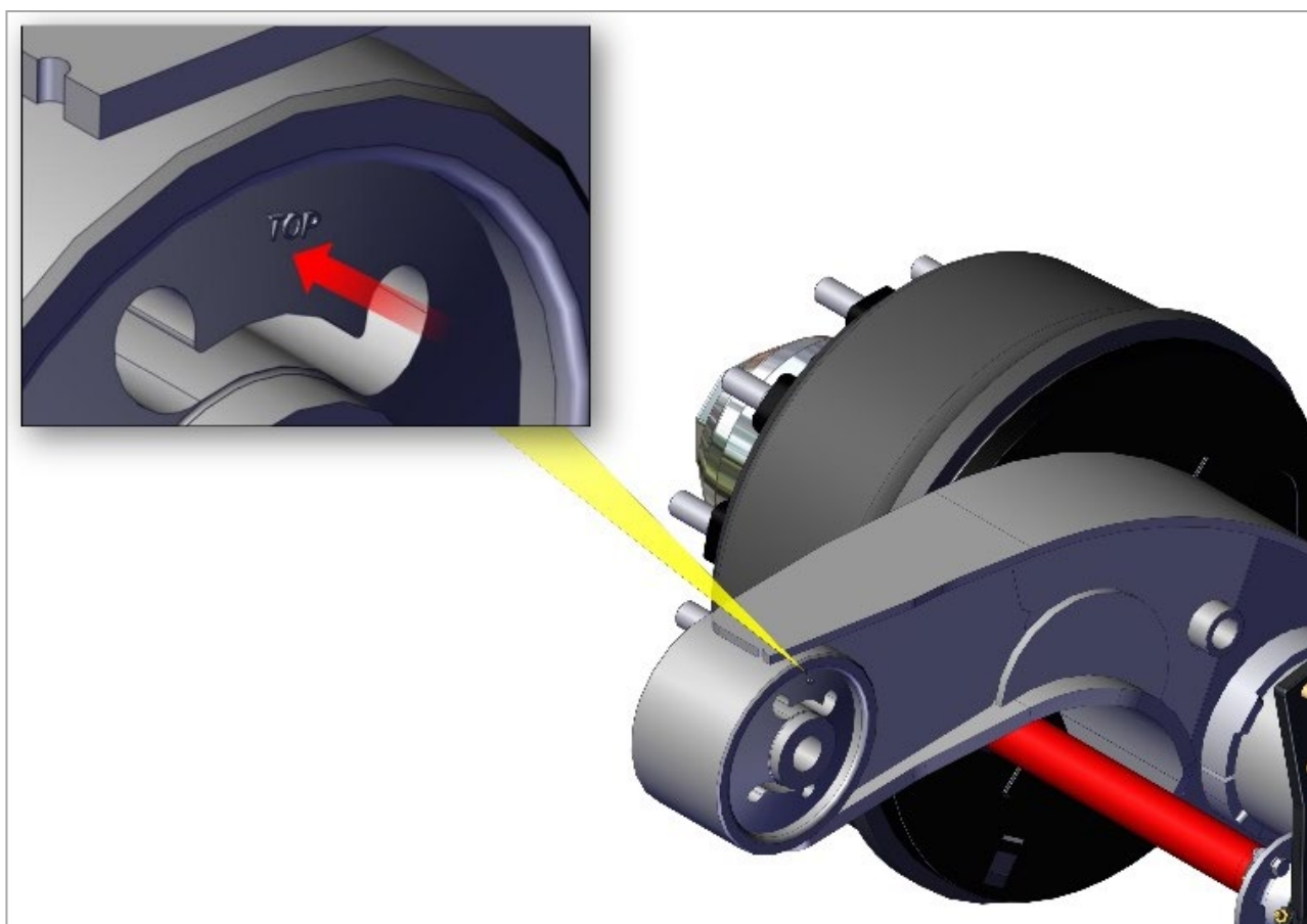
Рис. 7. Установка сайлентблока.
