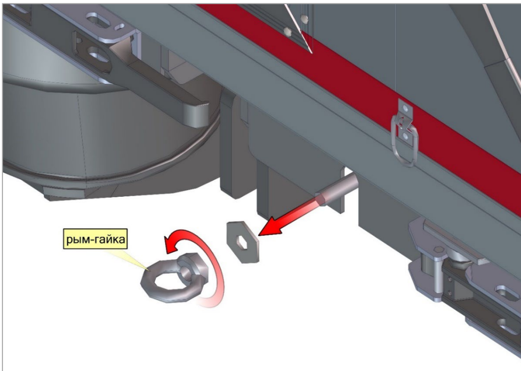
Рис. 37.2. Снятие рым-гаек
