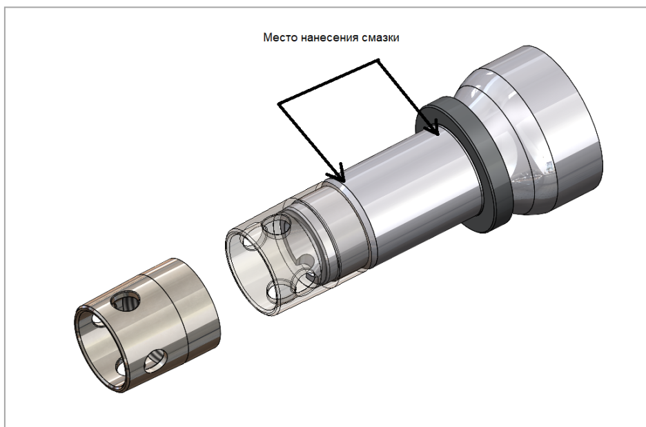
Рис. 10.1. Место нанесение смазки.
