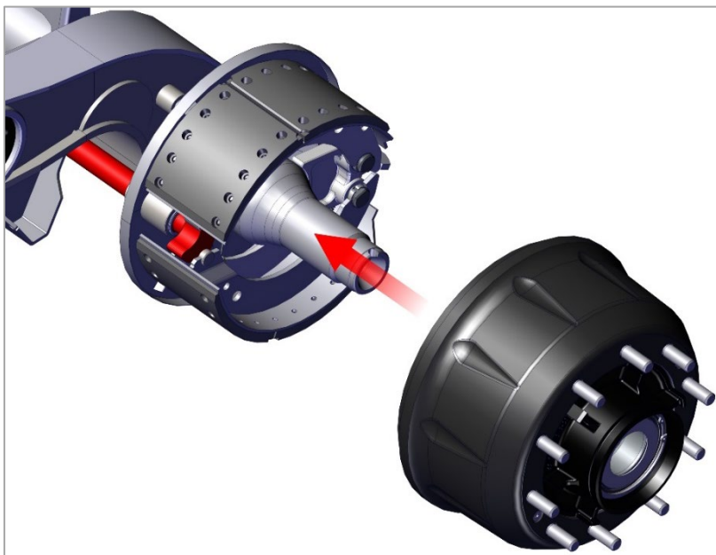
Рис. 14. Монтаж тормозного барабана.
