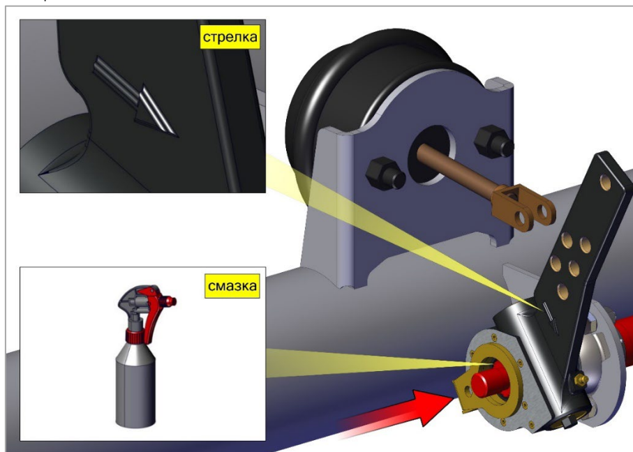
Рис. 23. Установка регулятора.
