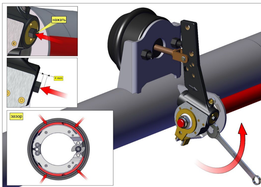
Рис. 23.8. Фиксатор.
