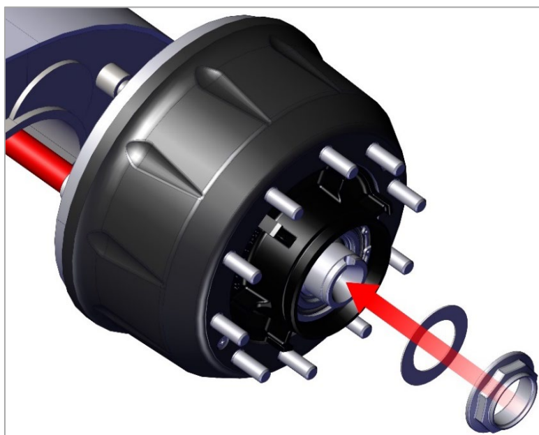
Рис. 14.1. Монтаж упорной шайбы и гайки подшипников ступицы.
