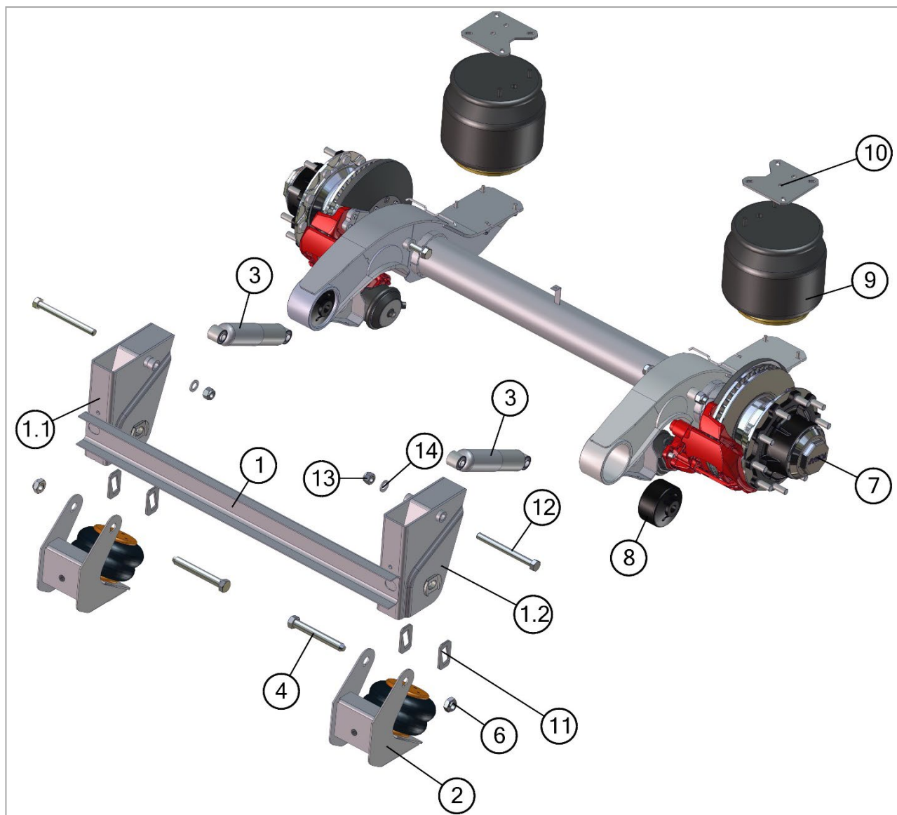
Рис. 6. Взрыв-схема рычажной подвески с дисковыми тормозами.
