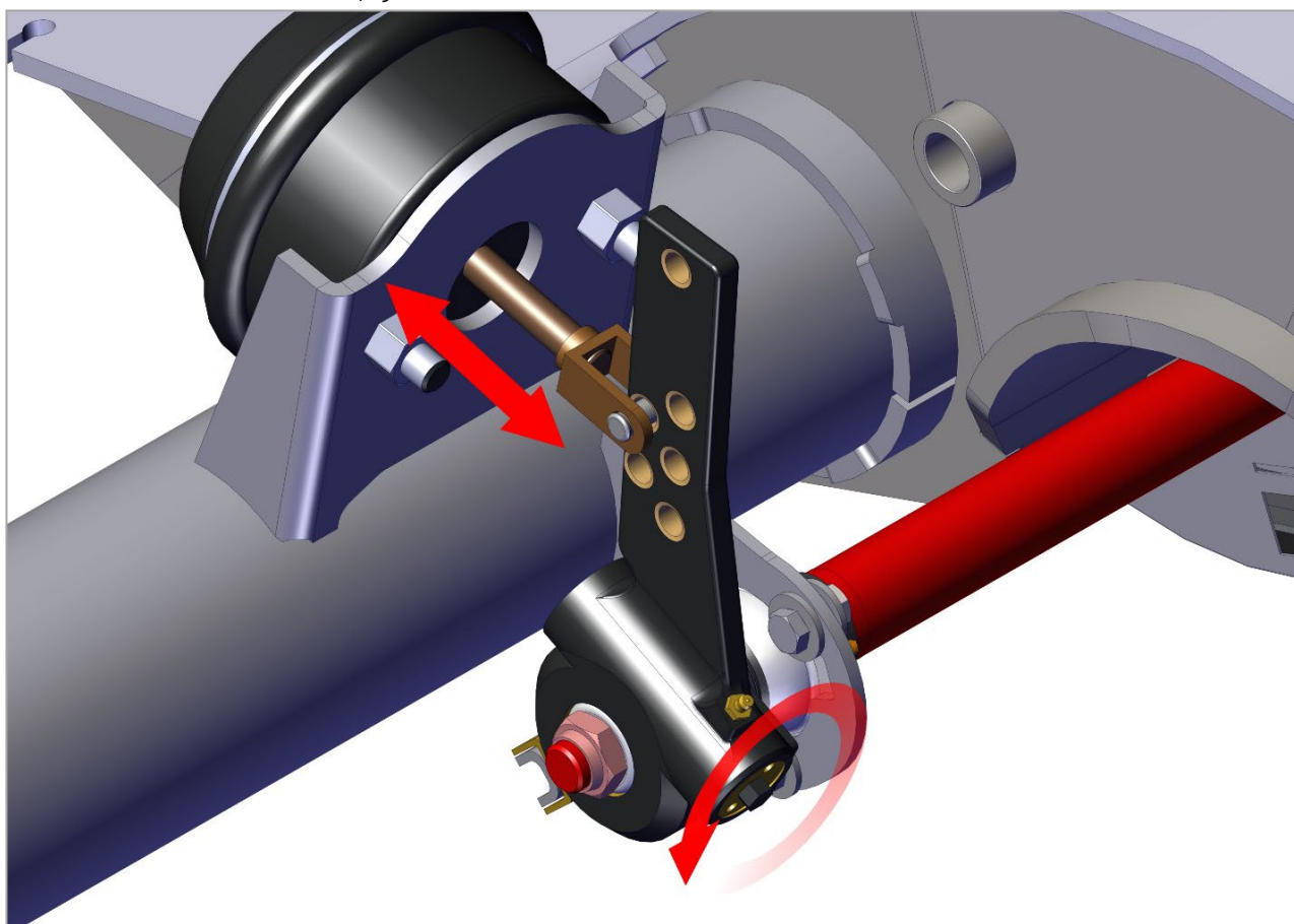
Рис. 24. Ход тормозной камеры.
