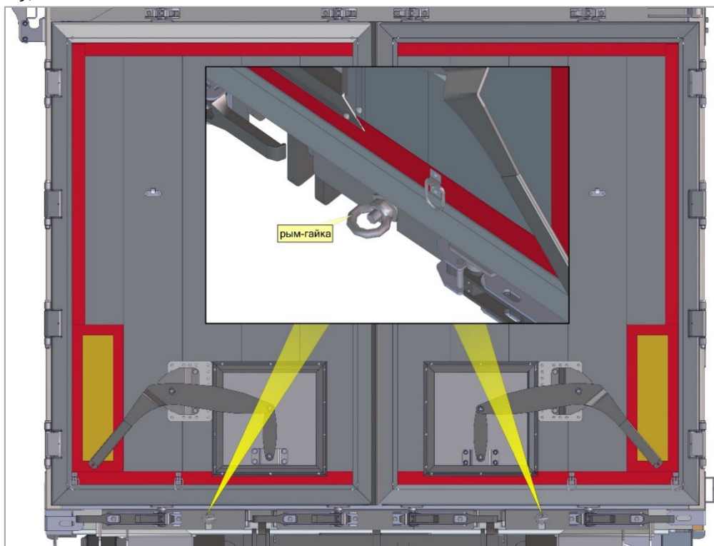
Рис. 40.2. Положение рым-гаек
