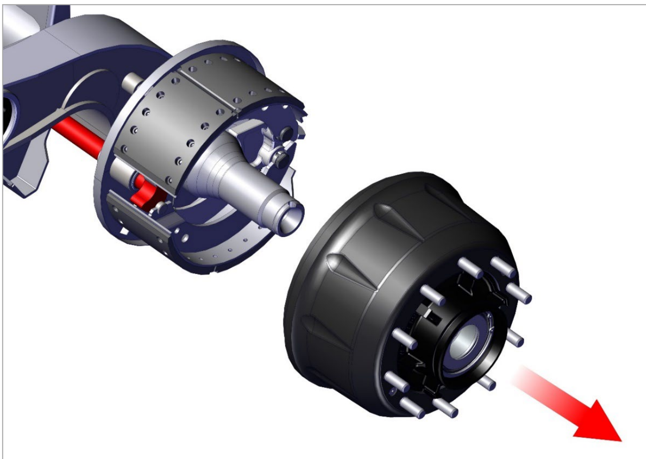
Рис. 12.1. Снятие сборочного узла ступицы и барабана.
