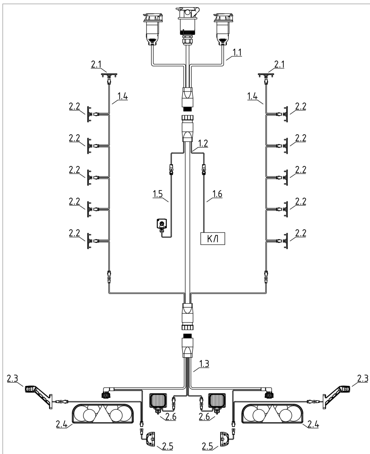
Рис. 34. Схема электрооборудования
