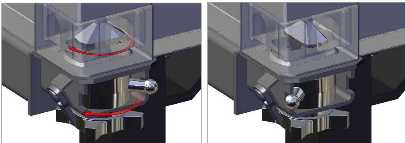
Рис. 82, 83. Фиксация передних стопоров контейнера
