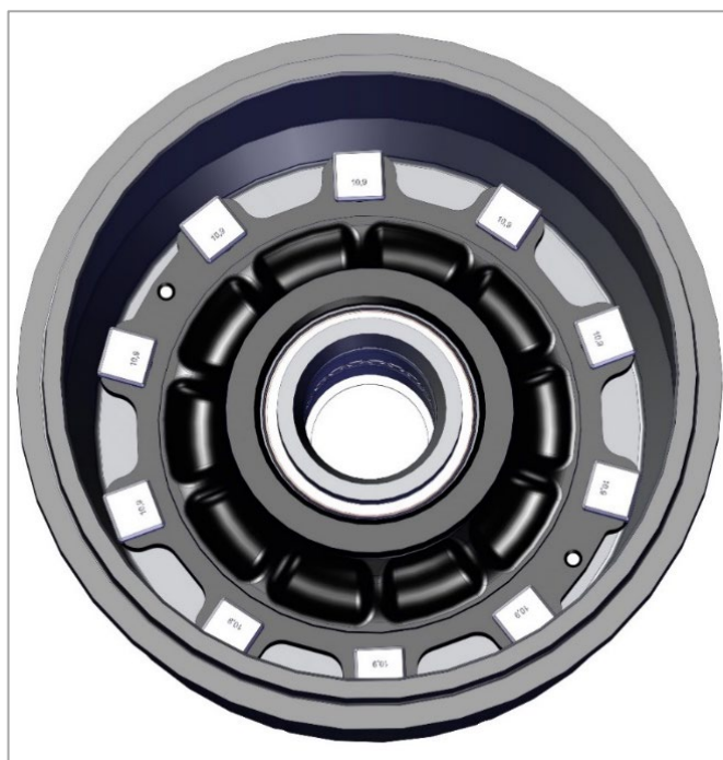
Рис. 14. Внешний вид барабана (внутренняя часть)
