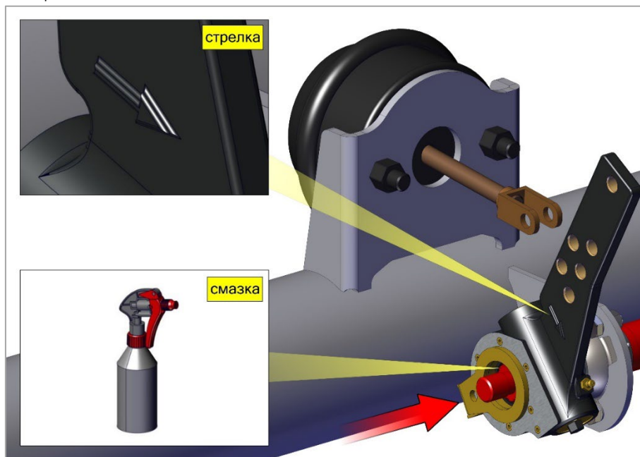
Рис. 30. Установка регулятора.
