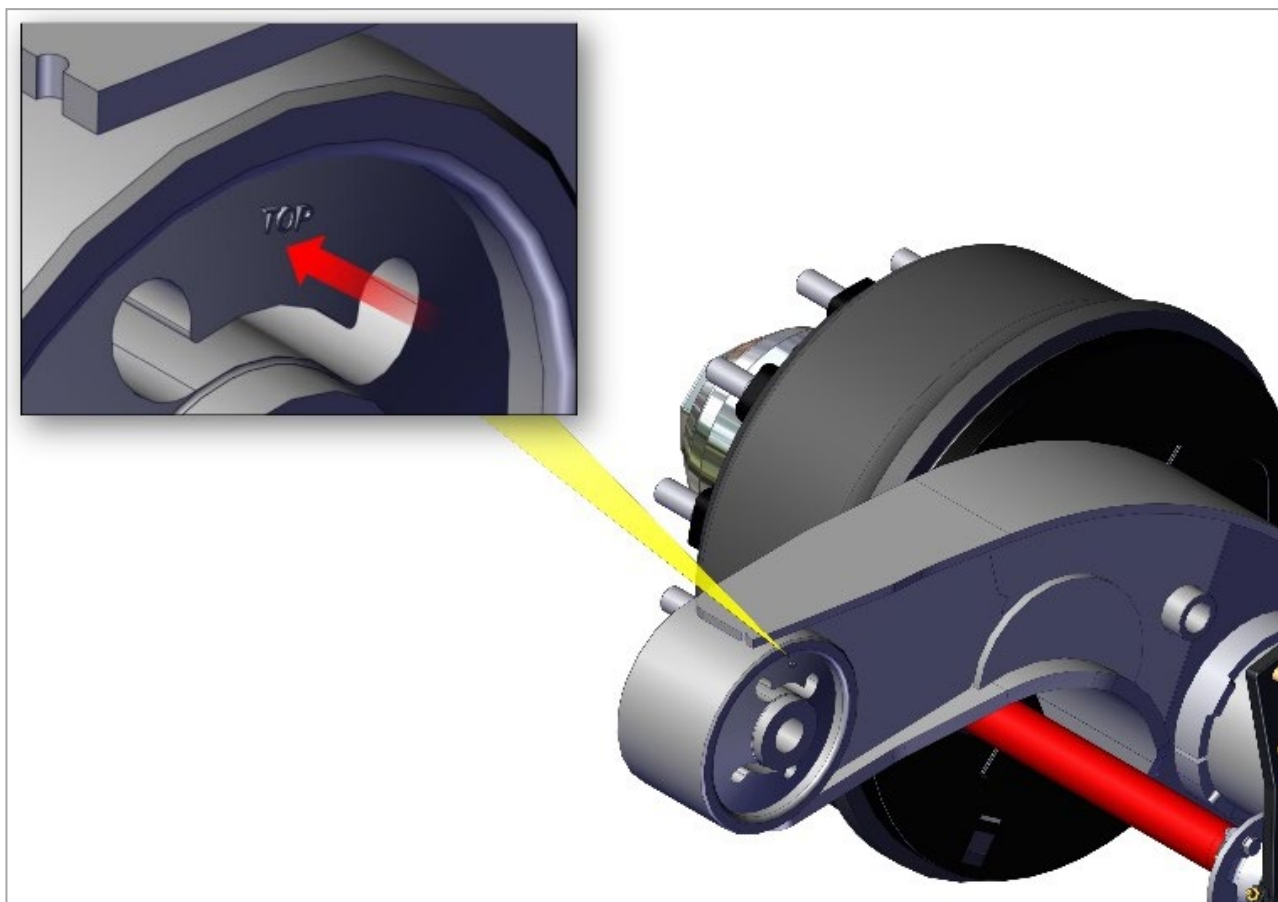
Рис. 6. Установка сайлентблока.
