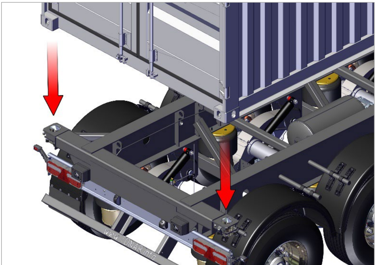
Рис. 78 Установка контейнера
