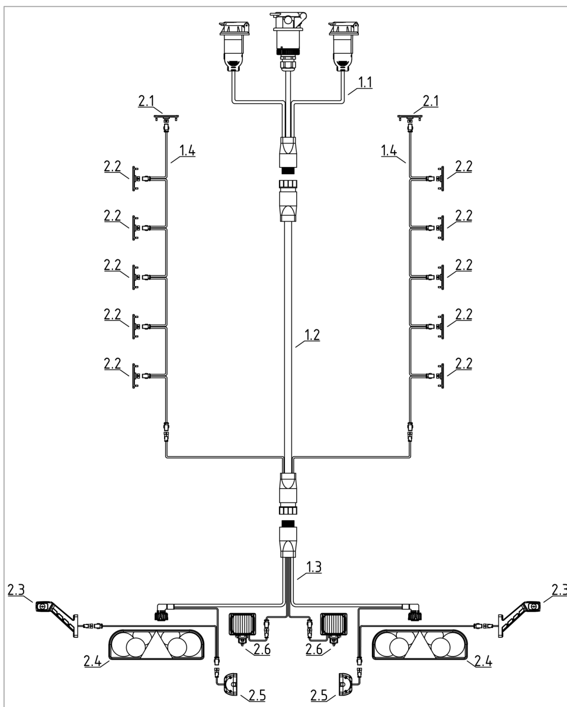
Рис. 62. Схема устройства электрооборудования
