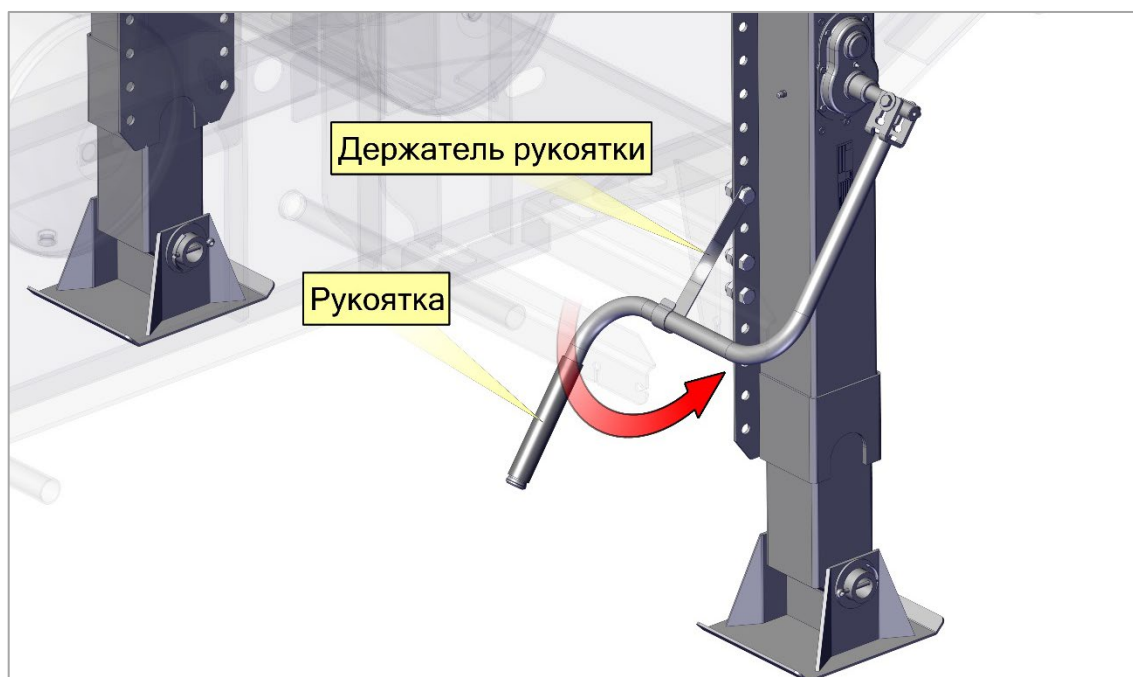
Рис.64, Достать рукоятку
