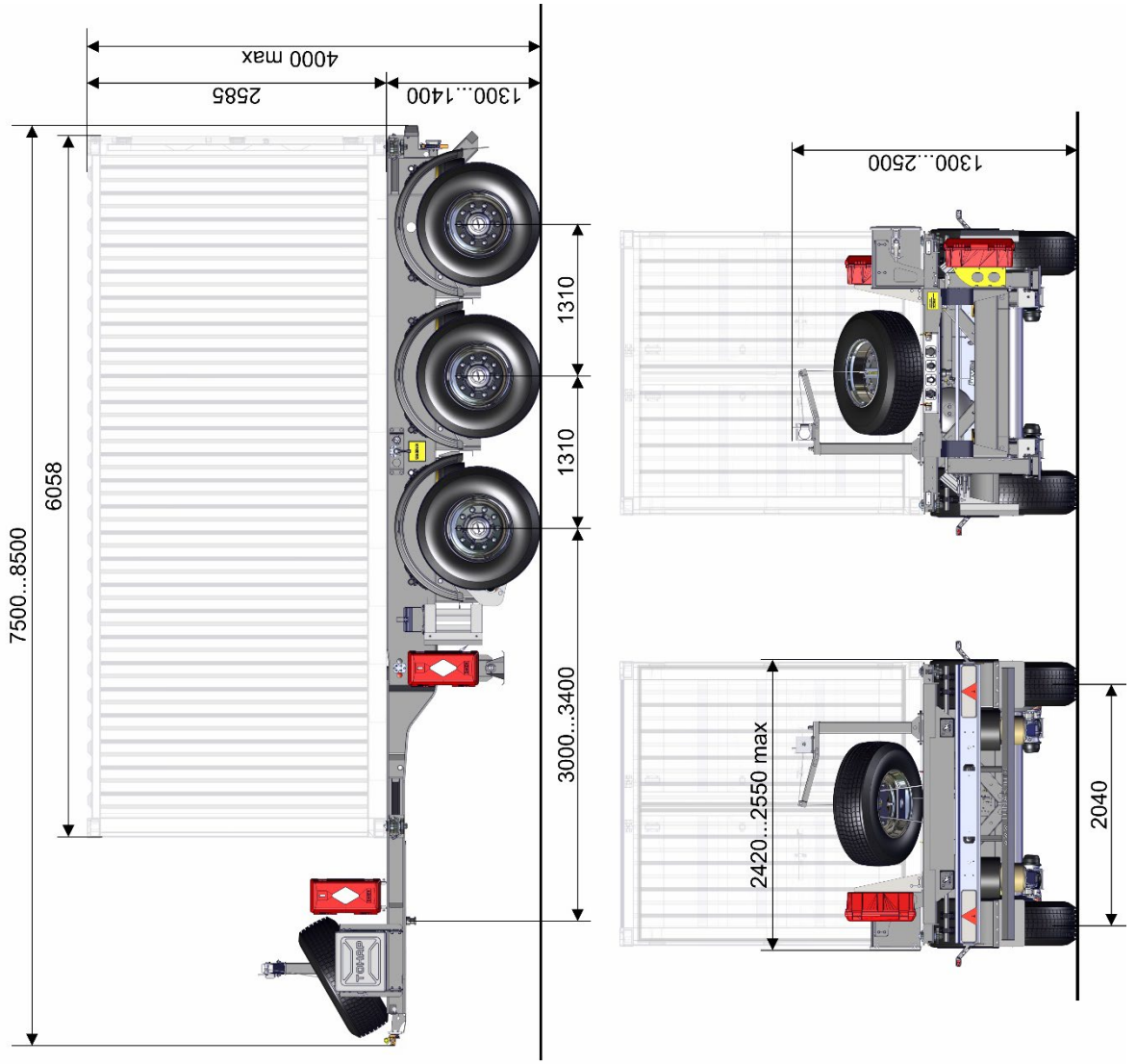
Рис.86. Габаритный чертёж модели 99886.
