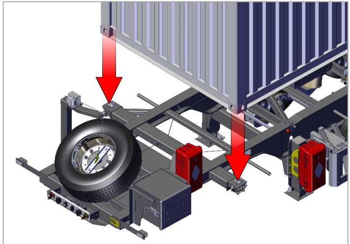
Рис. 80 Установка контейнера
