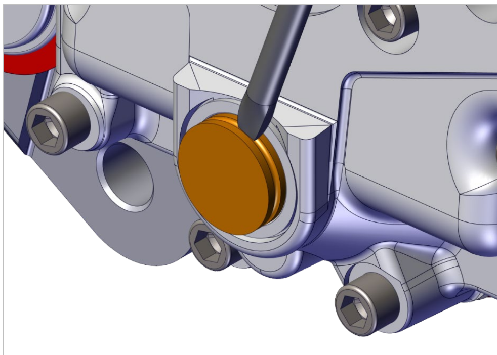
Рис. 48. Извлечение заглушки.
