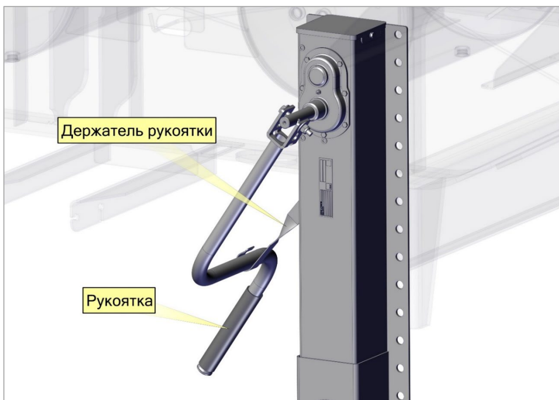
Рис.66, Положение рукоятки в фиксаторе
