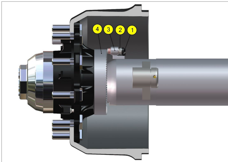
Рис. 8. Датчики ABS
