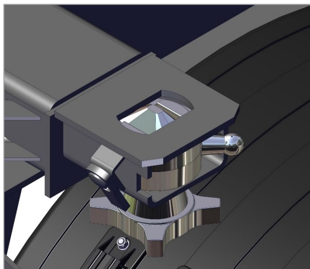
Рис. 76. Рис. 77. Положение стопоров контейнера
