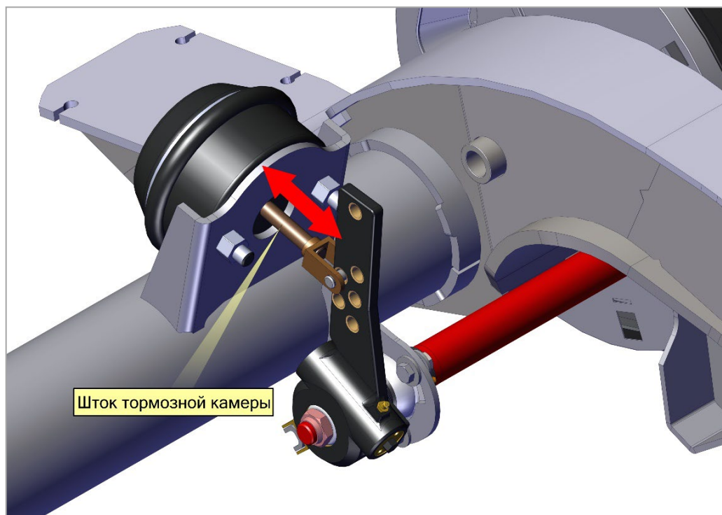
Рис. 29. Шток тормозных камер.
