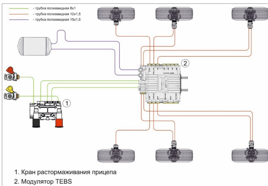
Рис. 57. Тормозной контур
