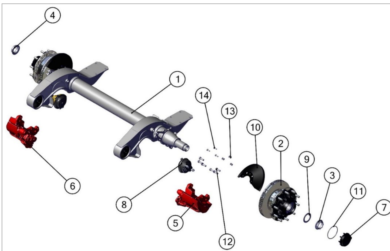
Рис. 40. Взрыв-схема оси с дисковыми тормозами.
