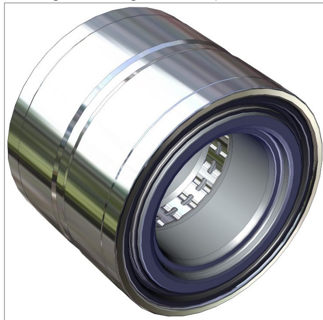
Рис. 17. Блок-подшипник.
