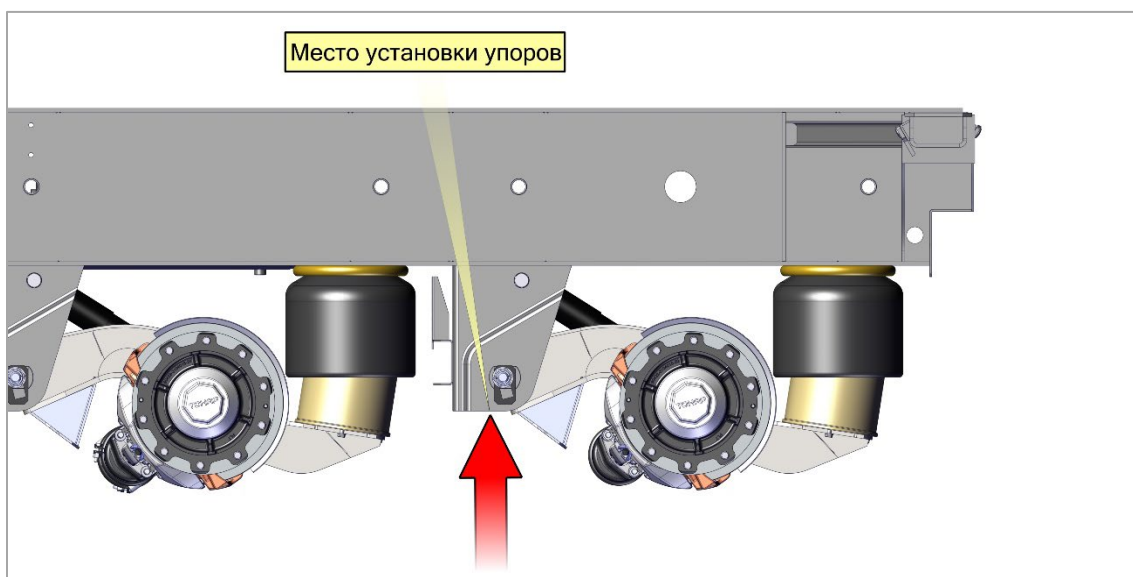
Рис. 42. Место установки упоров.
