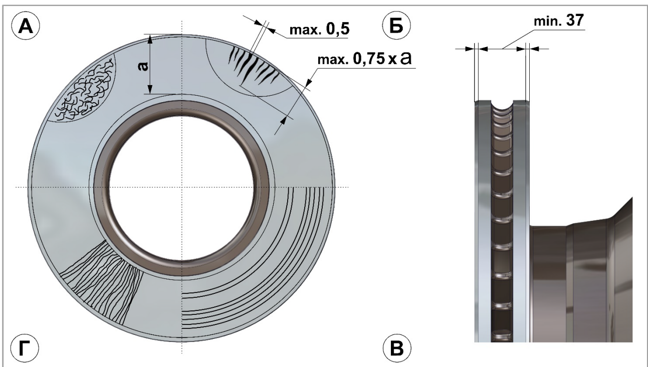
Рис. 52. Состояние рабочих поверхностей
