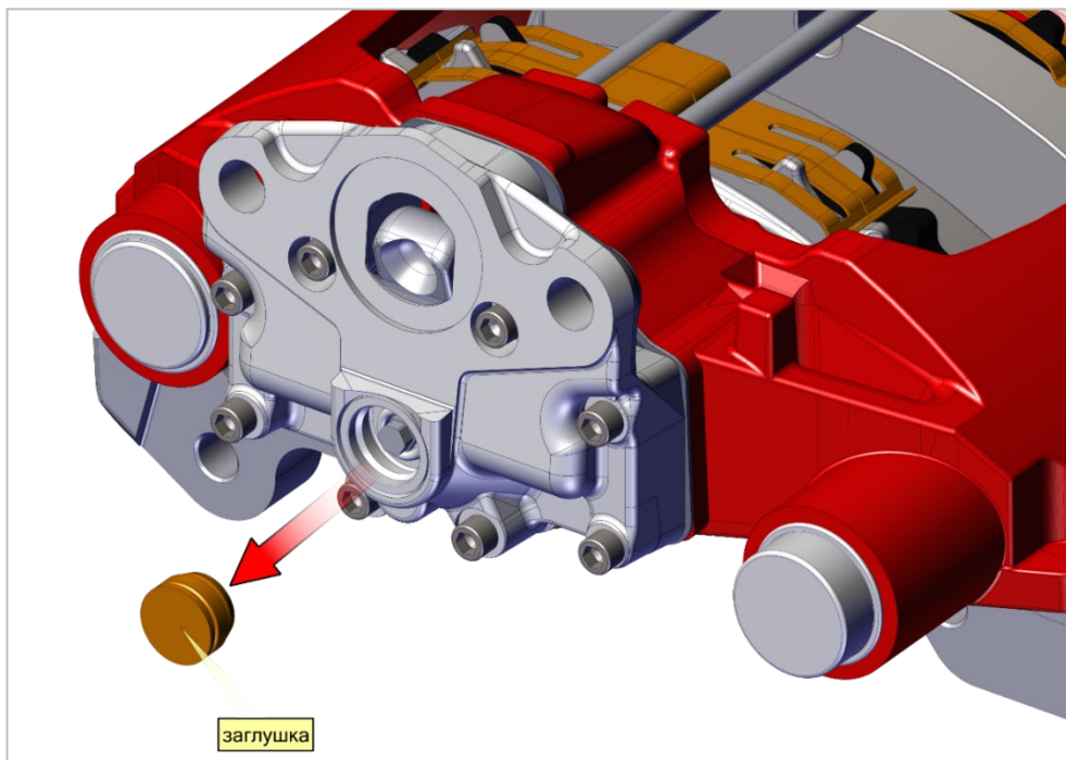
Рис. 47. Заглушка
