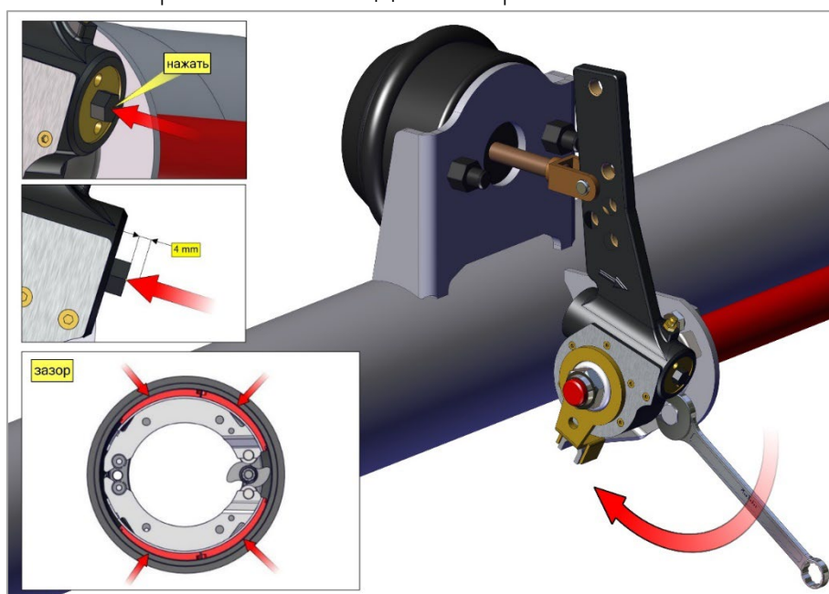
Рис.37. Фиксатор.
