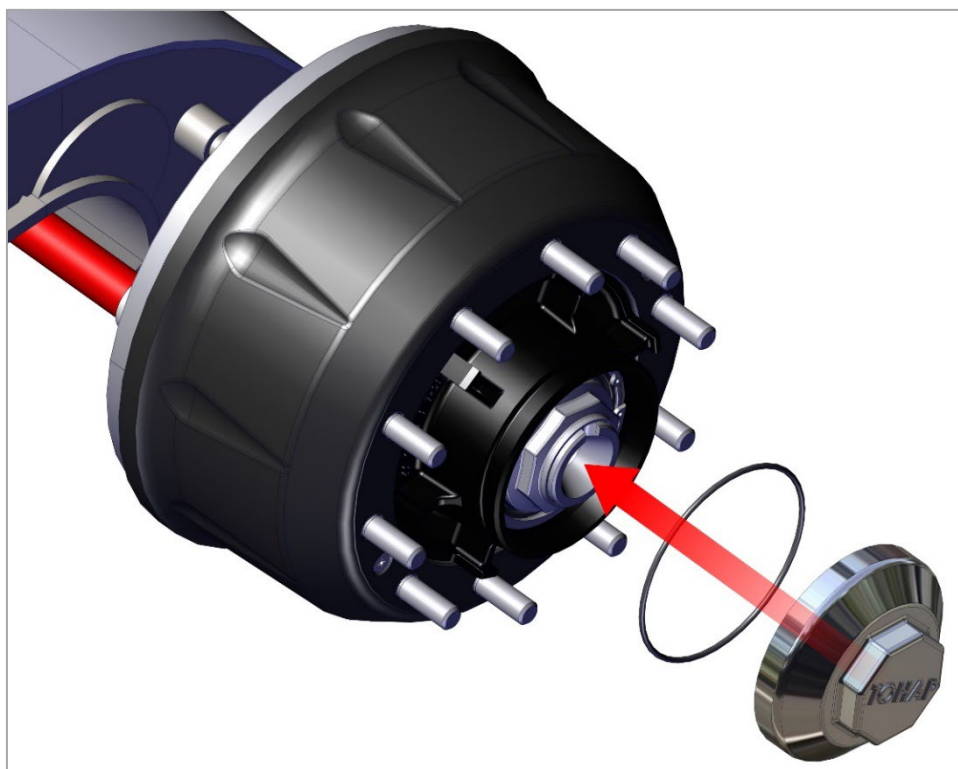
Рис. 21. Монтаж крышки ступицы колеса с резиновым уплотнительным кольцом.
