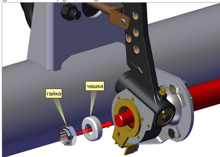
Рис.33. Закрепить регулятор.
