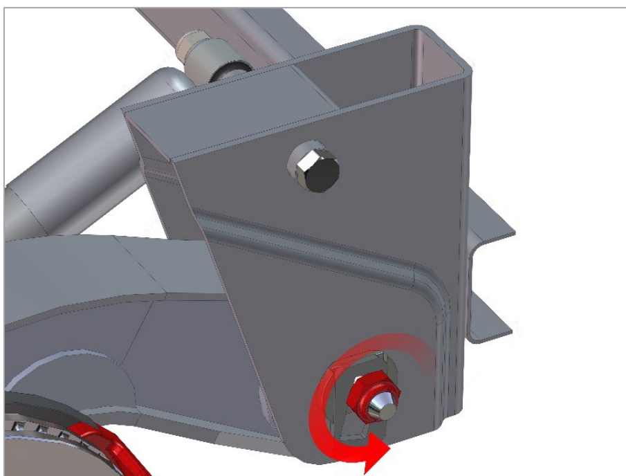
Рис. 44. Гайки рессорного болта.
