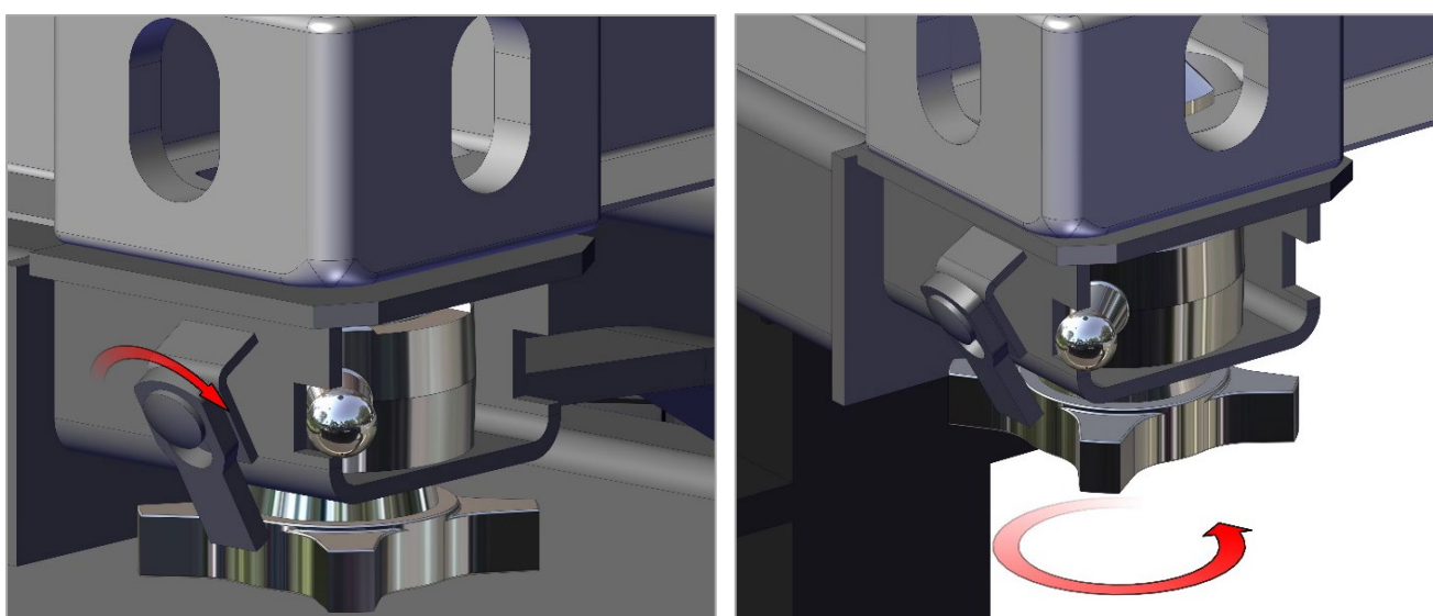
Рис. 82, 83. Фиксация передних стопоров контейнера
