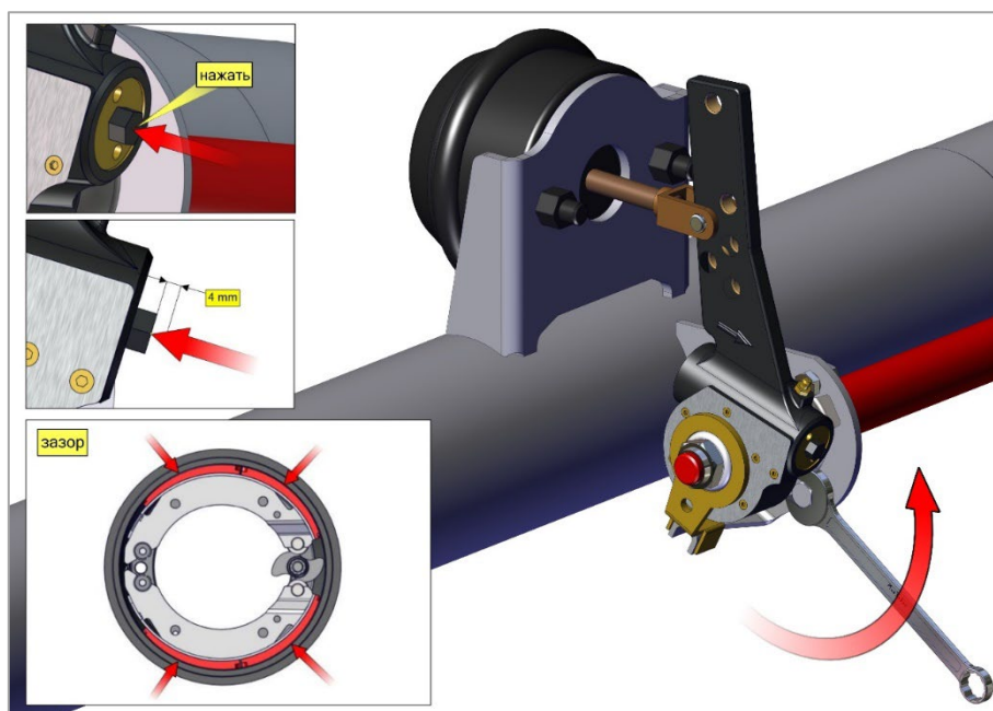
Рис. 38. Фиксатор.
