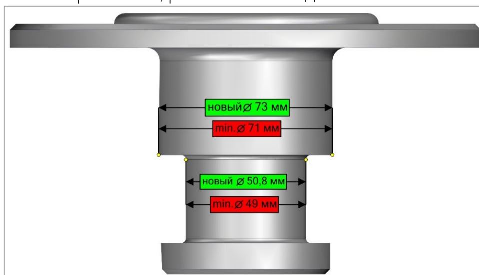
Рис. 74. Шкворень.
