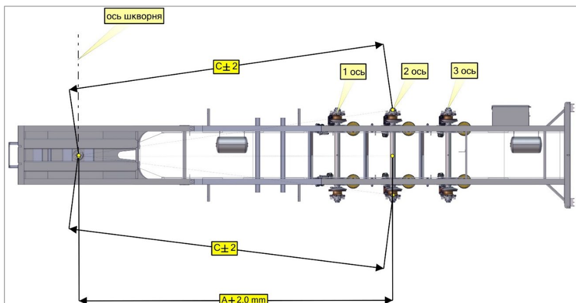
Рис. 46. Регулировка осей.
