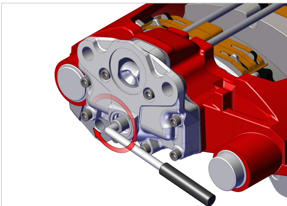
Рис. 50. Регулировка зазора.
