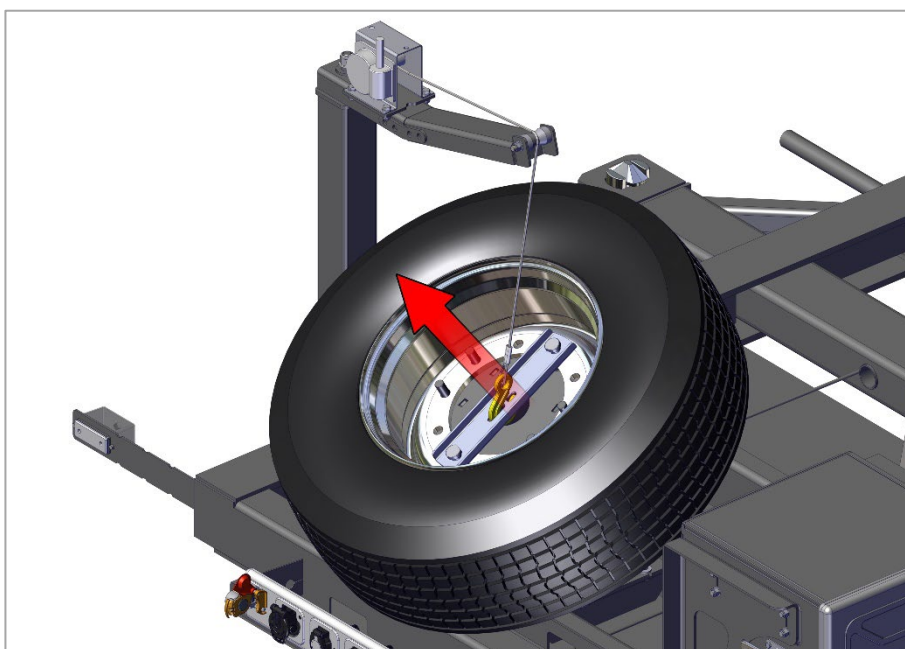
Рис. 70. Снятие колеса
