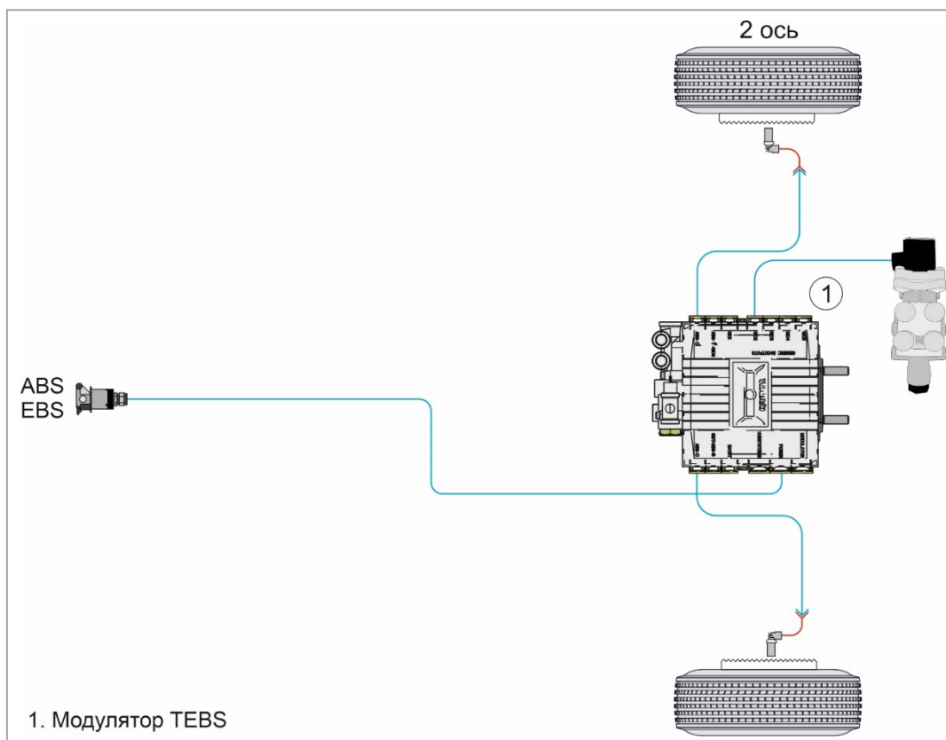
Рис. 58. Электрическая схема
