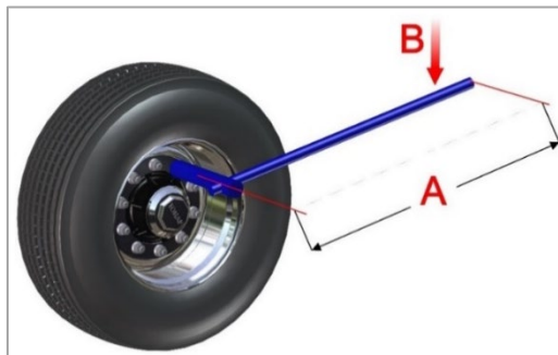
Рис. 55. Затяжка гаек
