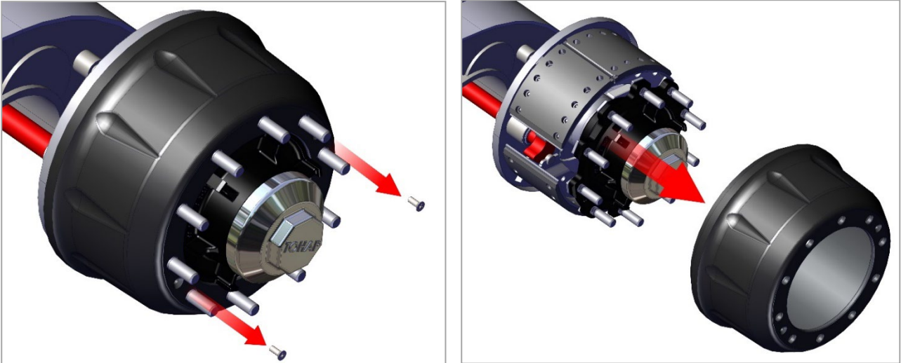
Рис. 15. и рис. 16. Снятие барабана.
