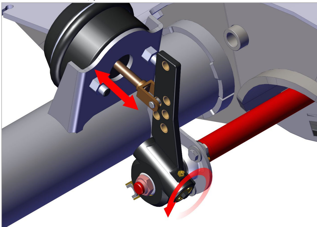
Рис. 39. Ход тормозной камеры.
