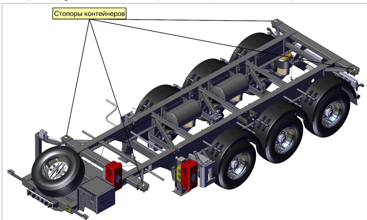
Рис. 1. Стопоры контейнера.
