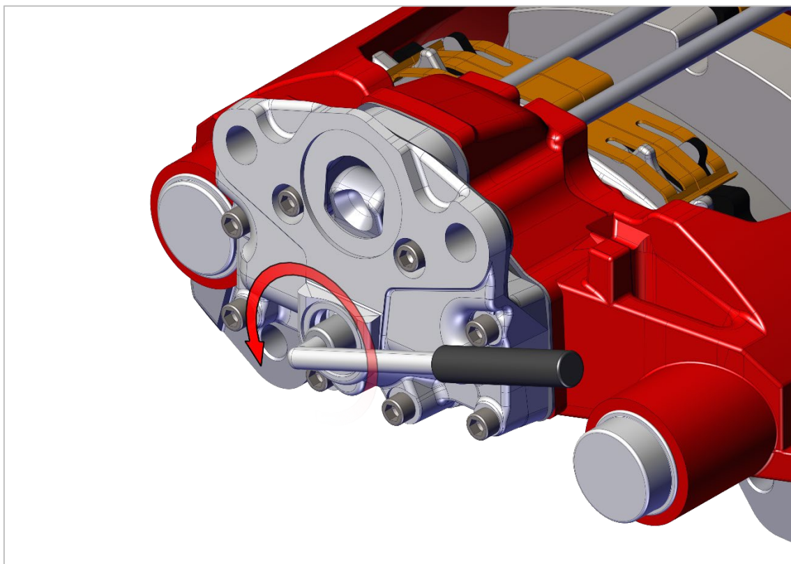
Рис. 51. Регулировка зазора.
