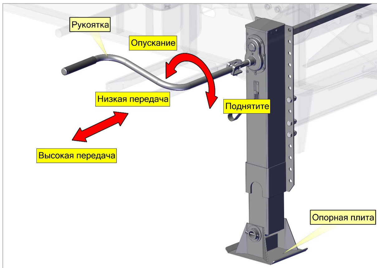
Рис.65, Управление опорным устройством
