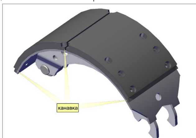
Рис. 24. Тормозная накладка.
