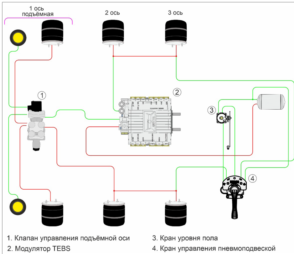
Рис. 56. Контур пневмоподвески
