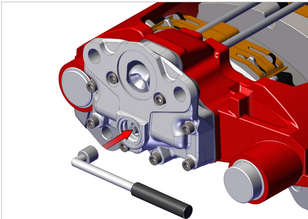
Рис. 49. Установка ключа.
