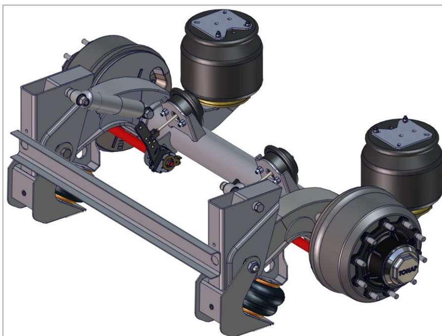
Рис. 2. Рычажная подвеска с барабанными тормозами.
