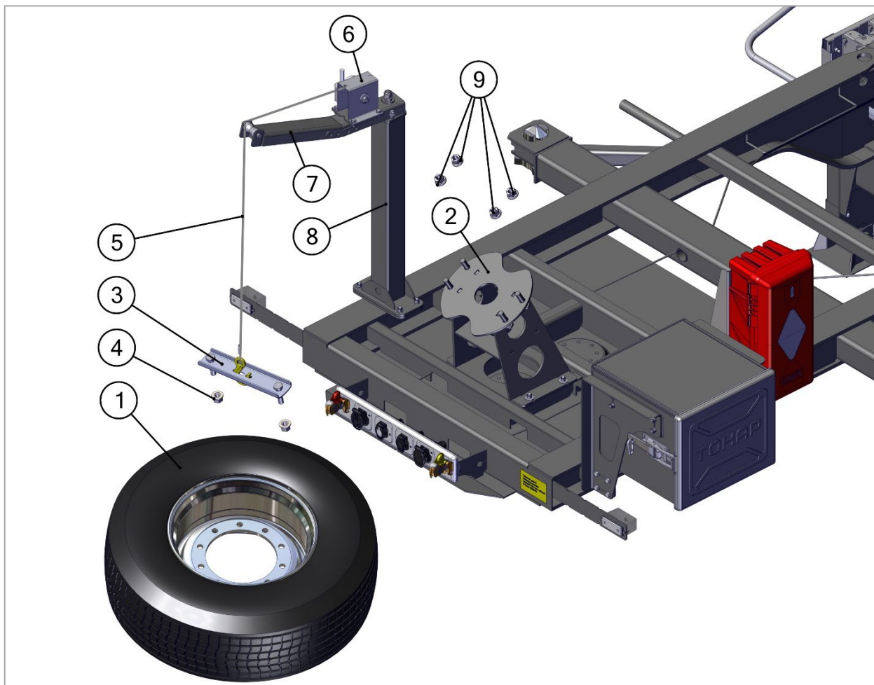
Рис. 67. Установка запасного колеса
