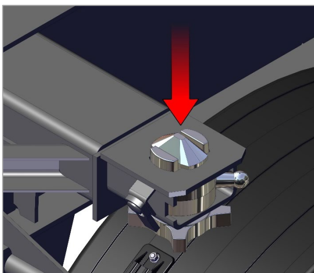
Рис. 76. Рис. 77. Положение стопоров контейнера
