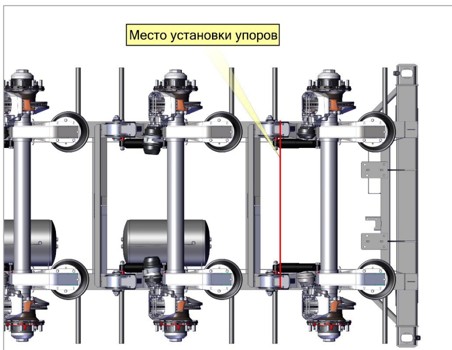
Рис. 43. Место установки упоров.
