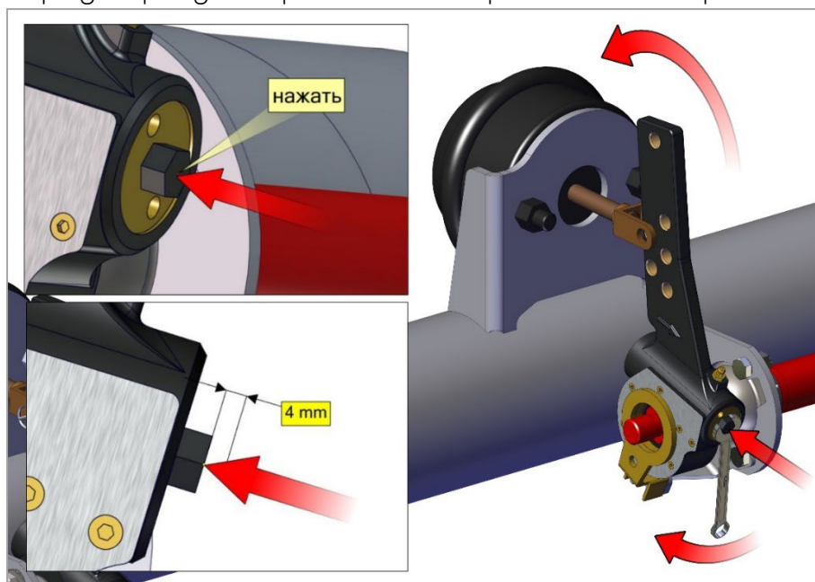
Рис. 31. Фиксатор.
