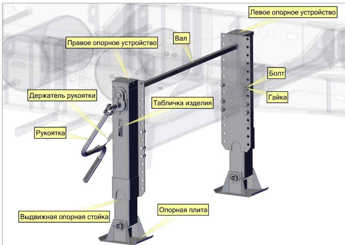
Рис. 63. Опорное устройство
