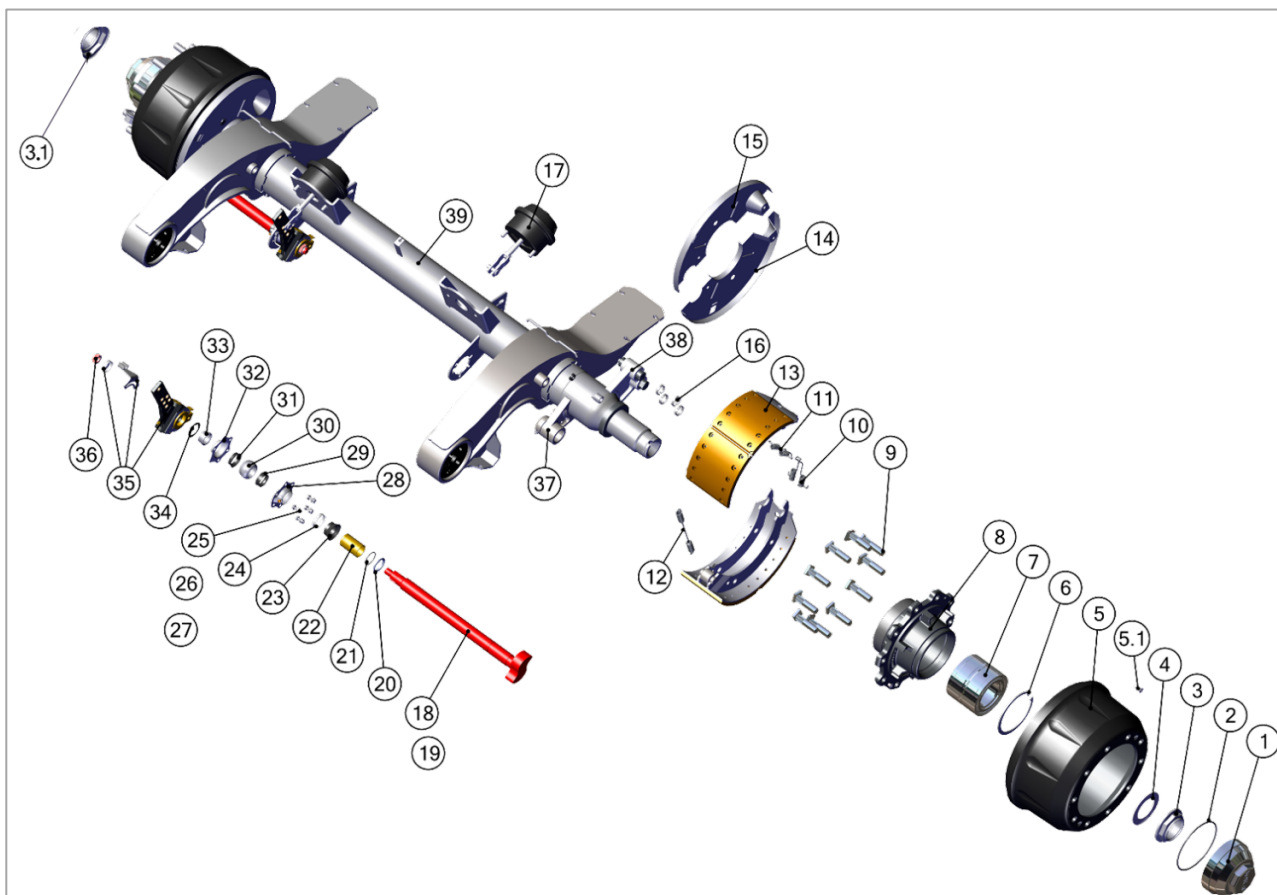
Рис. 6. Взрыв-схема оси полуприцепа с барабанными тормозами.
