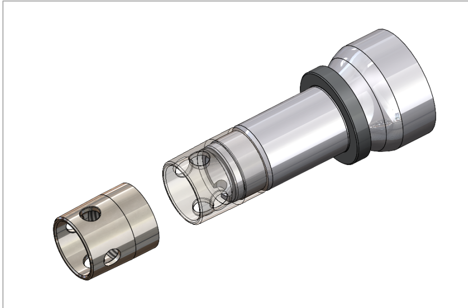
Рис. 8. Установка муфты защиты на резьбу цапфы.
