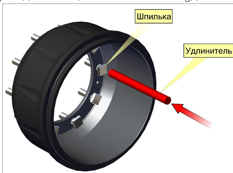
Рис. 14. Установка колесных шпилек.
