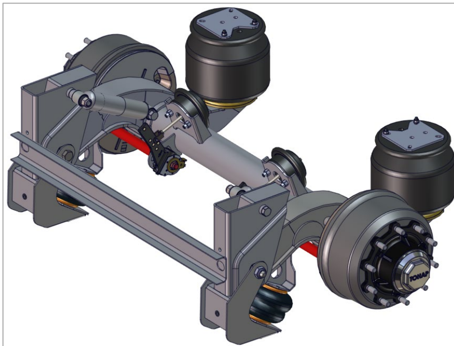
Рис. 1. Рычажная подвеска с барабанными тормозами.
