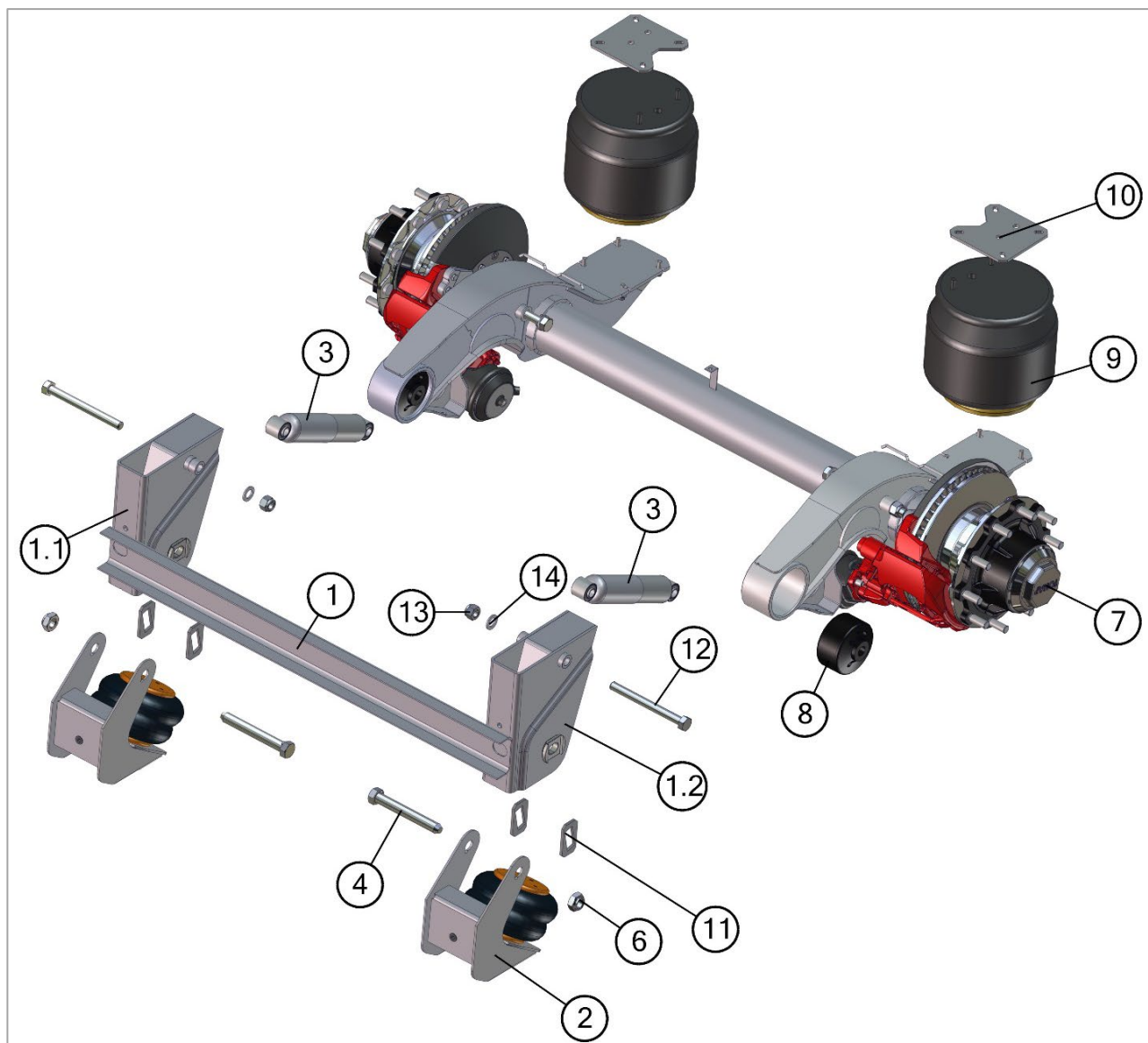
Рис. 4. Взрыв-схема рычажной подвески с дисковыми тормозами.
