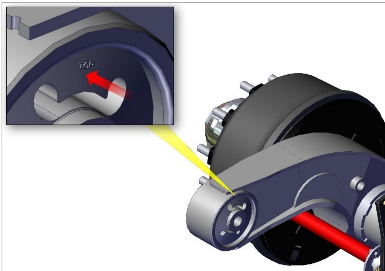
Рис. 5. Установка сайлентблока.
