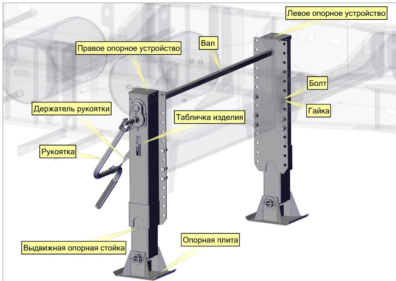
Рис. 31. Опорное устройство
