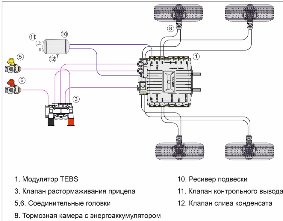
Рис. 29. Контур пневмоподвески
