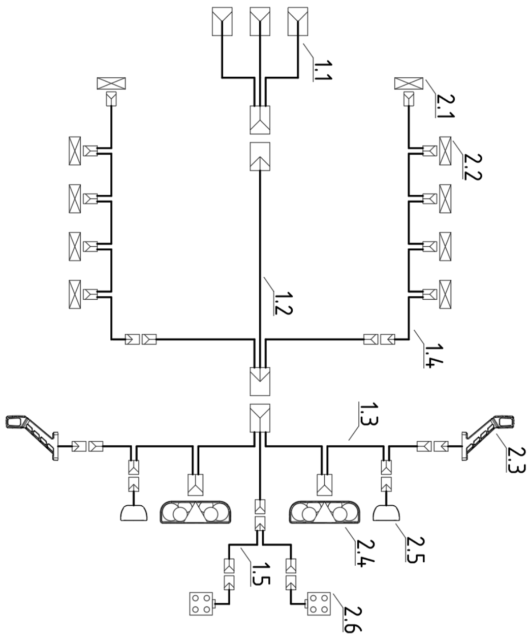
Рис. 32. Схема устройства электрооборудования
