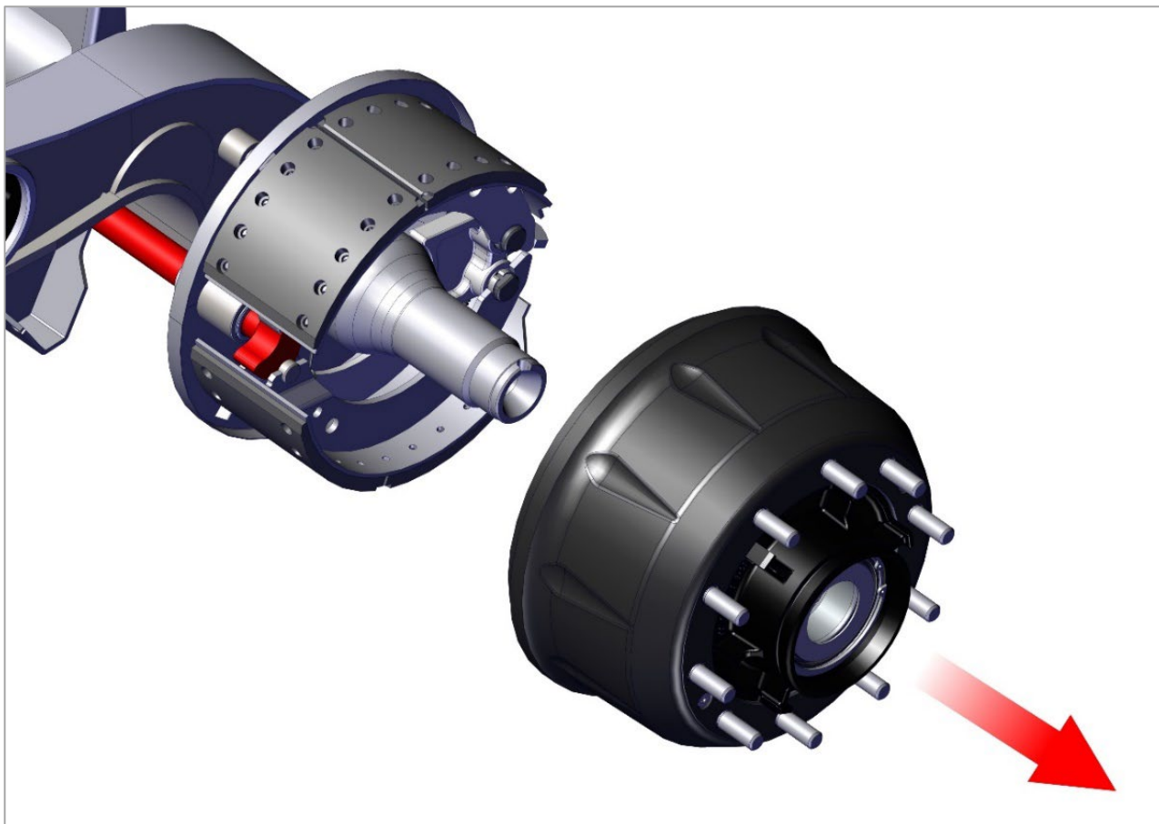
Рис. 10.1. Снятие сборочного узла ступицы и барабана.
