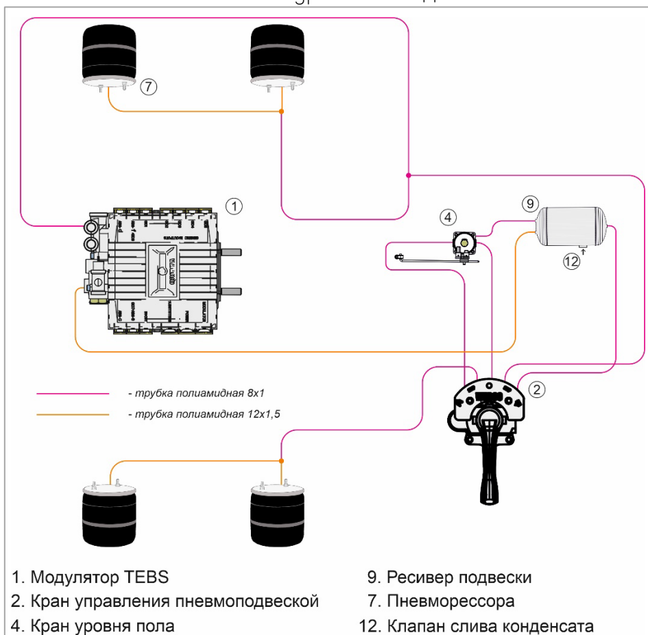
Рис. 29.1. Тормозной контур
