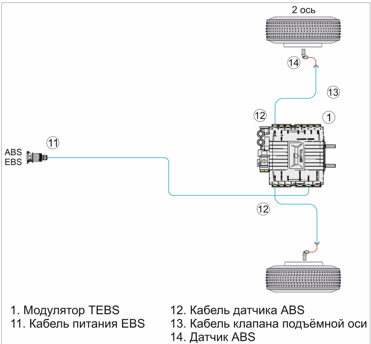
Рис. 29.2. Электрическая схема
