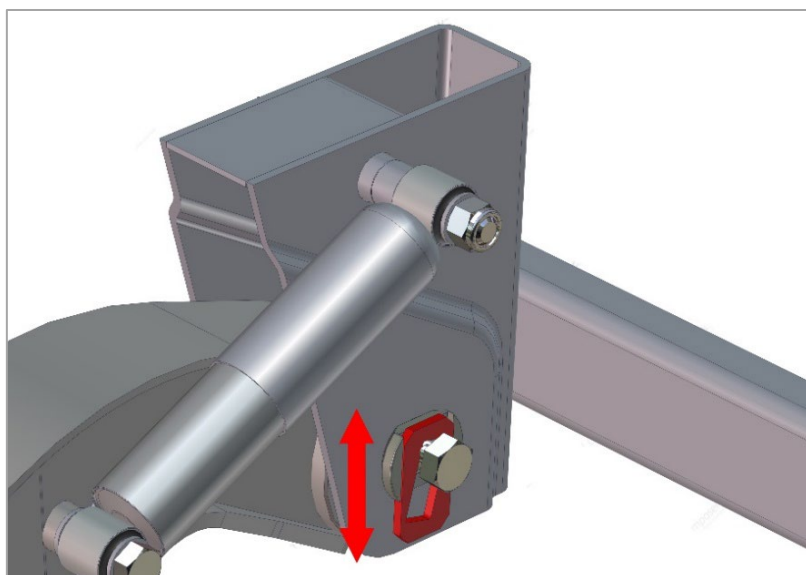
Рис. 25.1. Регулировочные пластины.
