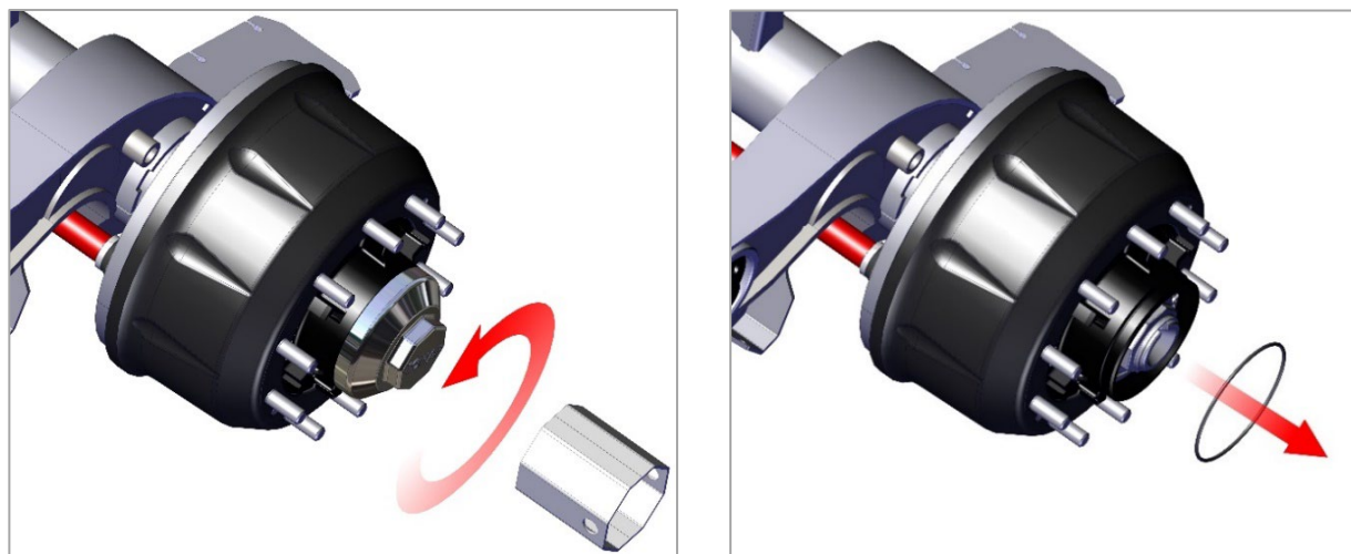
Рис. 9. Снятие крышки ступицы.
