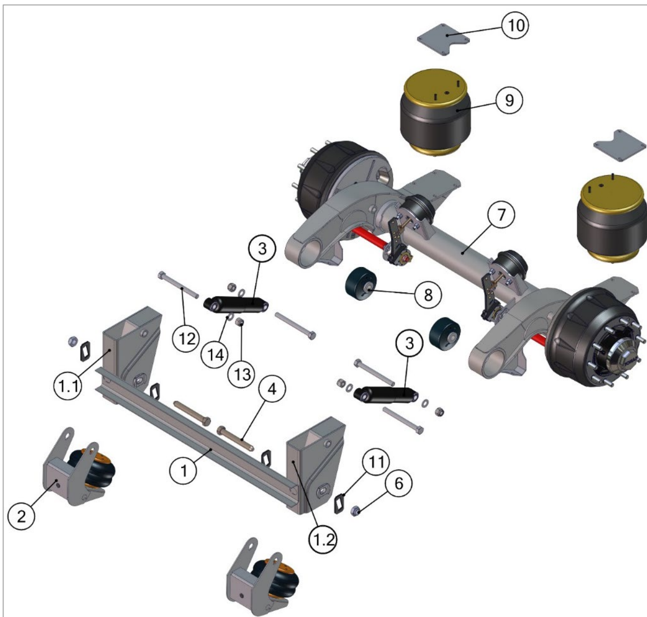
Рис. 3. Взрыв-схема рычажной подвески с барабанными тормозами.
