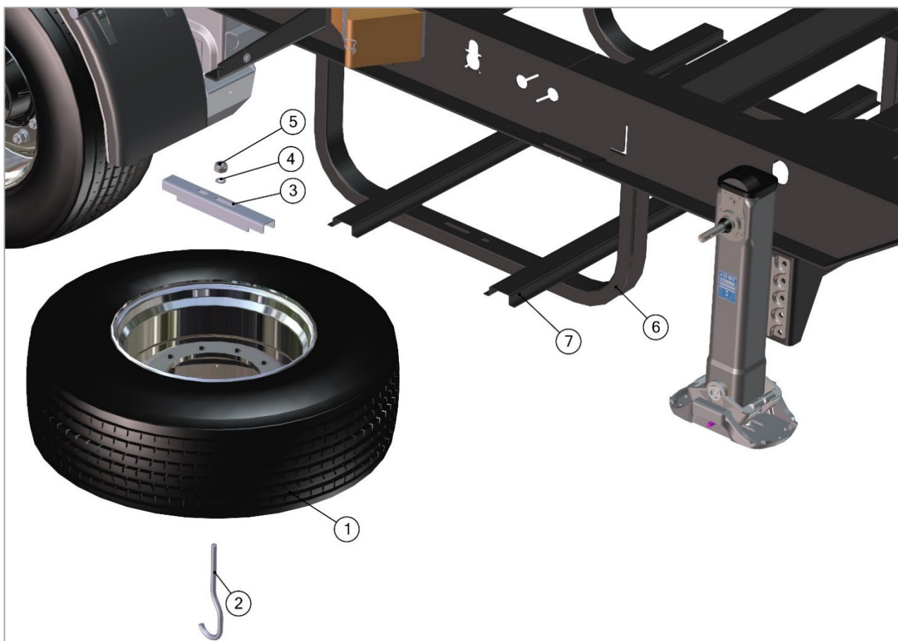
Рис. 33. Установка запасного колеса.
