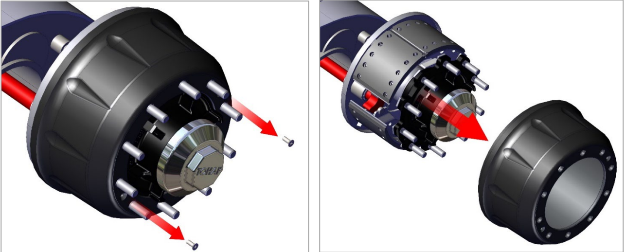
Рис. 10.2. и рис. 10.3. Снятие барабана.
