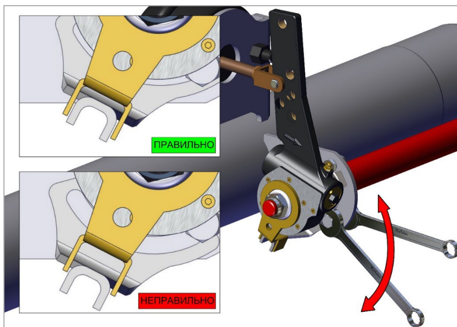
Рис. 21.6. Закрепить регулятор.
