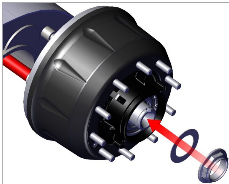
Рис. 12.1. Монтаж упорной шайбы и гайки подшипников ступицы.
