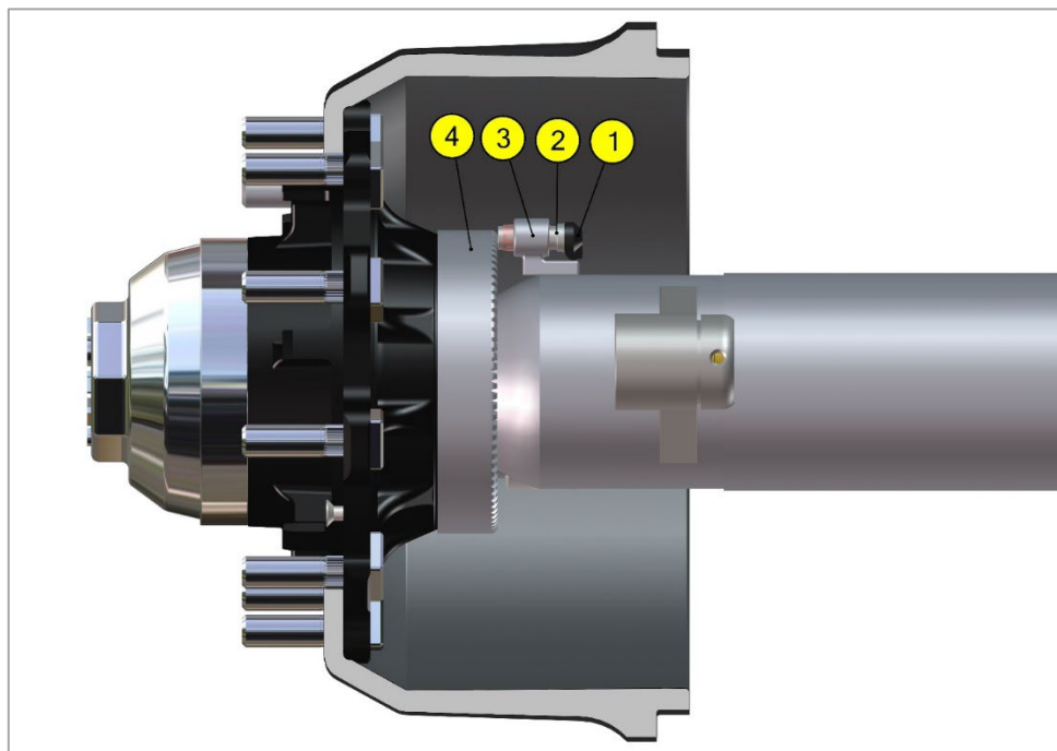
Рис. 7. Датчики ABS
