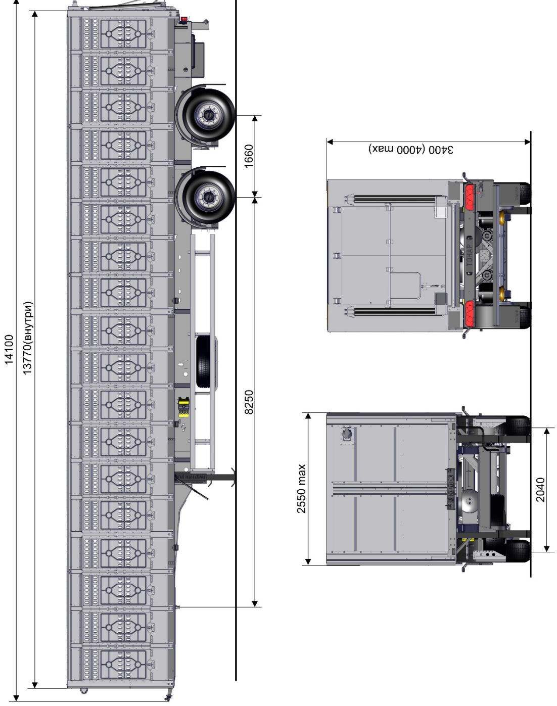
Рис. 36. Габаритный чертёж модели 98262.
