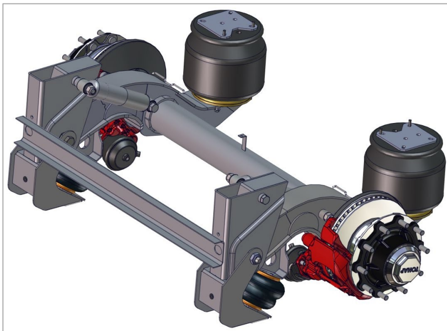
Рис. 2. Рычажная подвеска с дисковыми тормозами.
