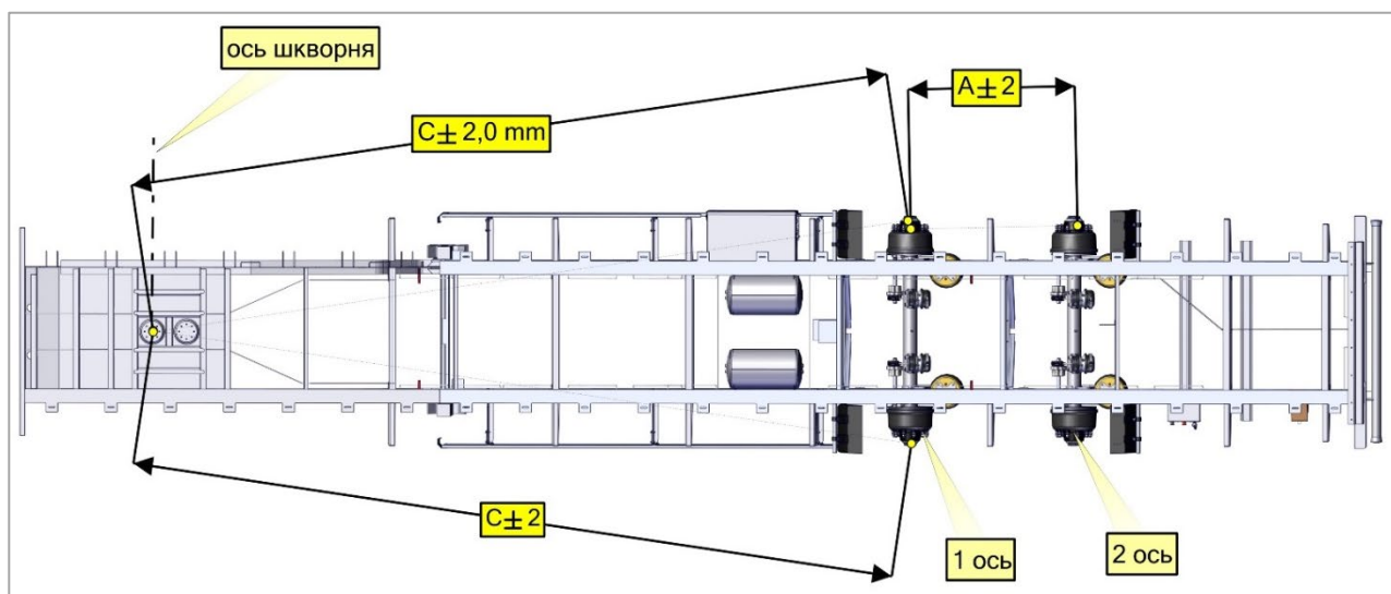
Рис. 25.2. Регулировка осей.
