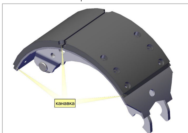
Рис. 15. Тормозная накладка.
