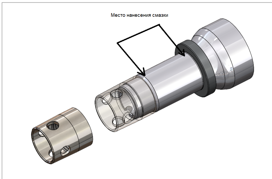
Рис. 8.1. Место нанесение смазки.
