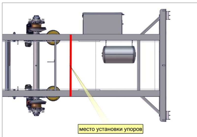
Рис. 24.2. Место установки упоров.
