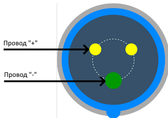
вид на розетку со стороны контактов
