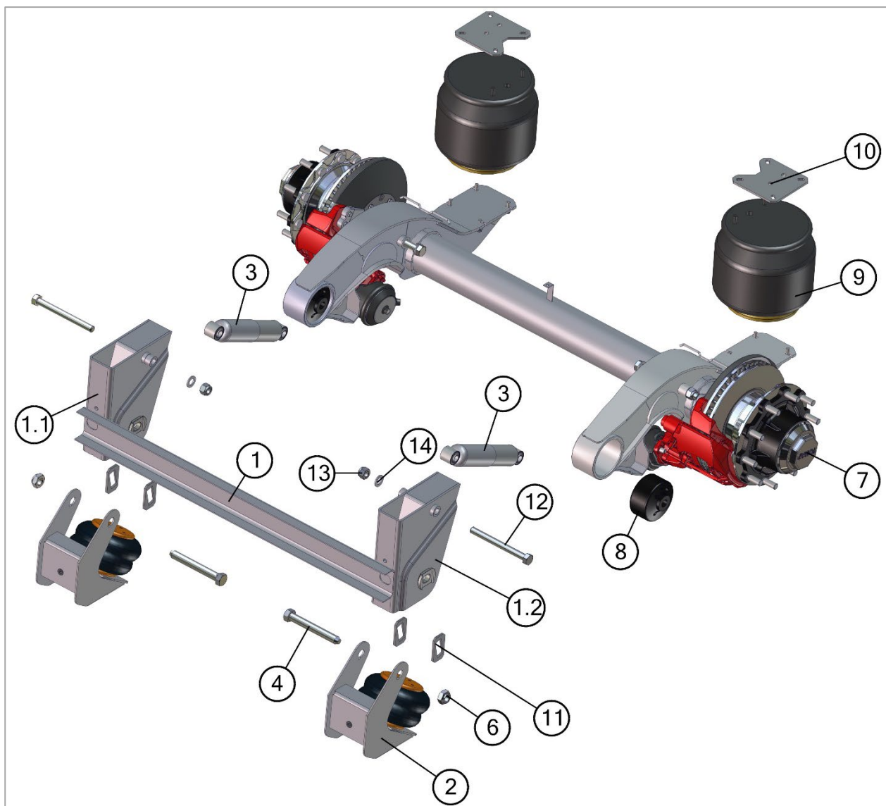
Рис. 8. Взрыв-схема рычажной подвески с дисковыми тормозами
