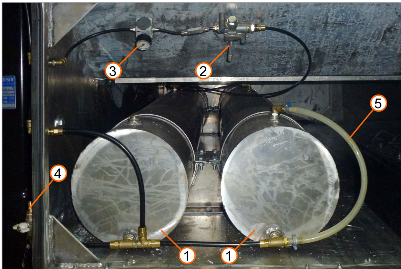
Рис.38. Система подачи воды
