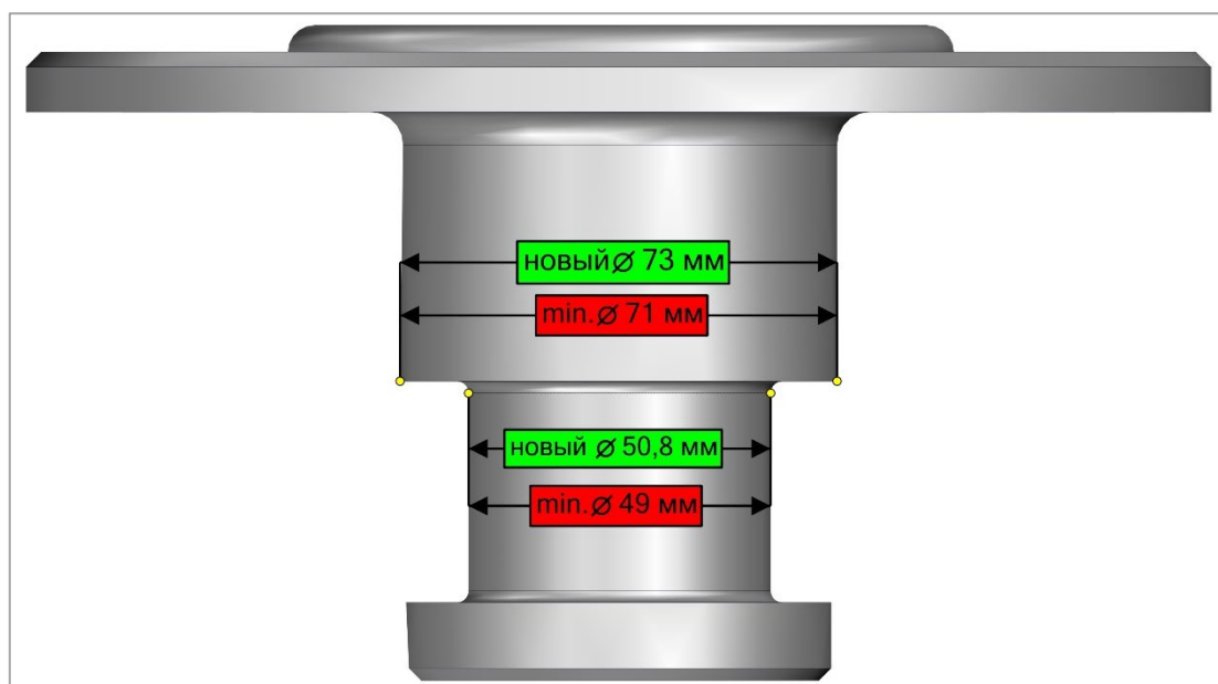
Рис. 31. Шкворень
