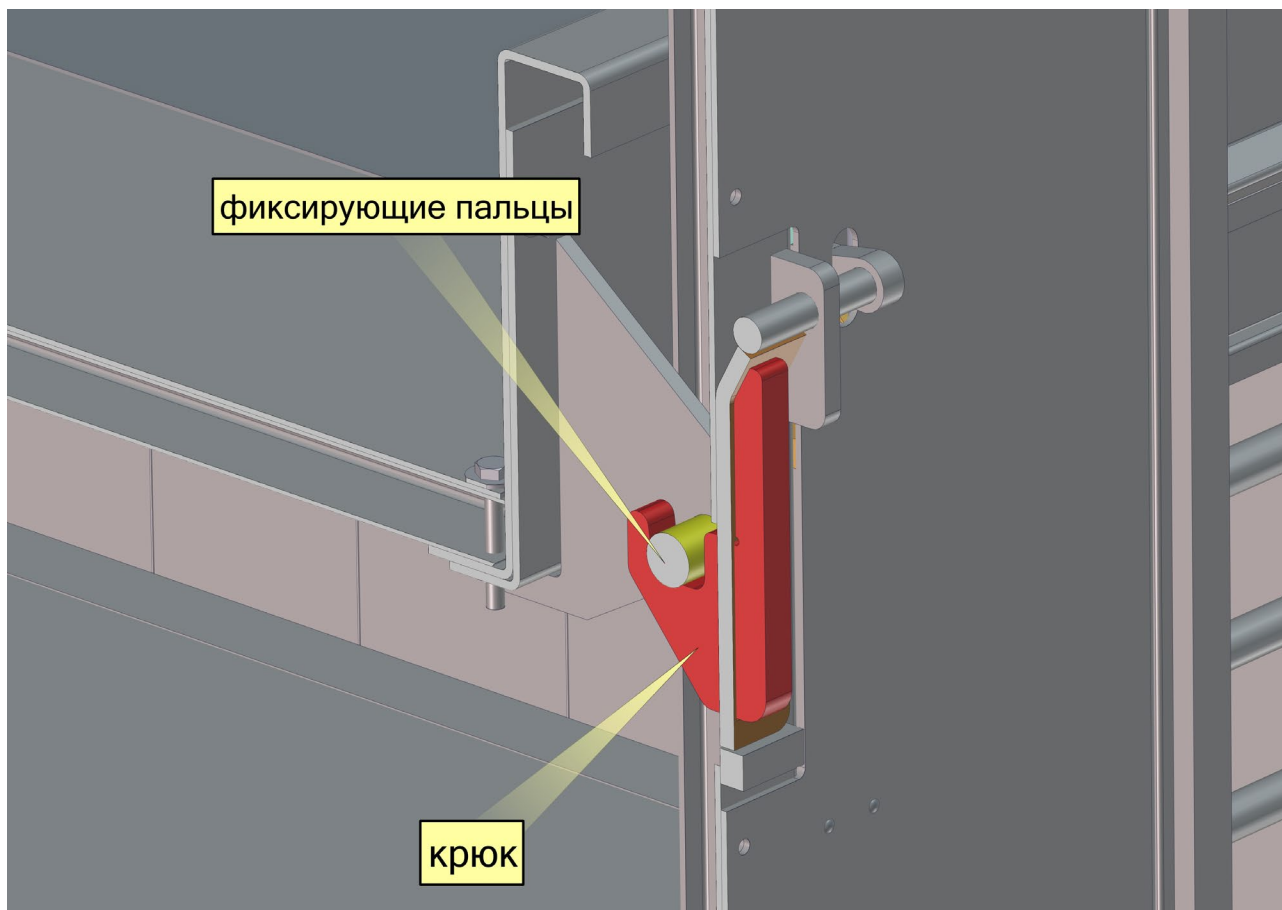
Рис. 37.1 Крюк и фиксирующий палец
