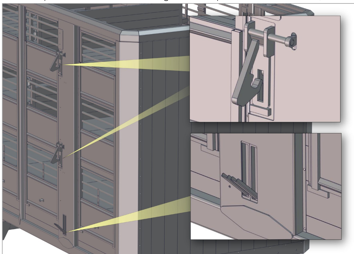
Рис 36. Положение замков привода и крюков
