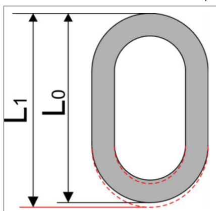
Рис. 34. Увеличение звена цепи
