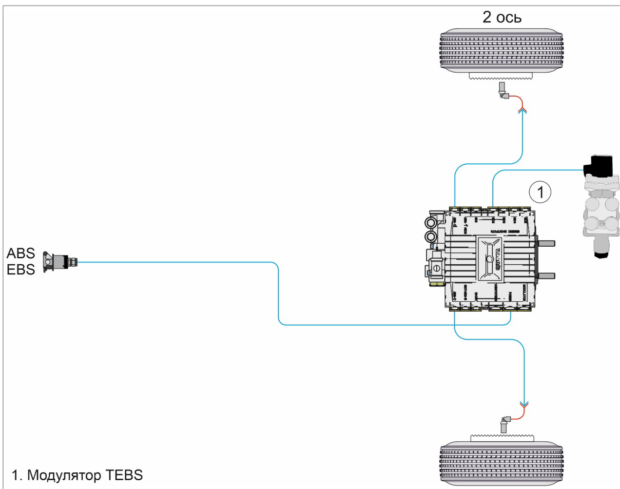
Рис. 29.2. Электрическая схема
