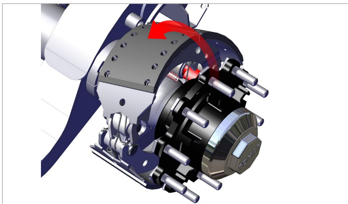
Рис. 19. Снятие тормозной колодки
