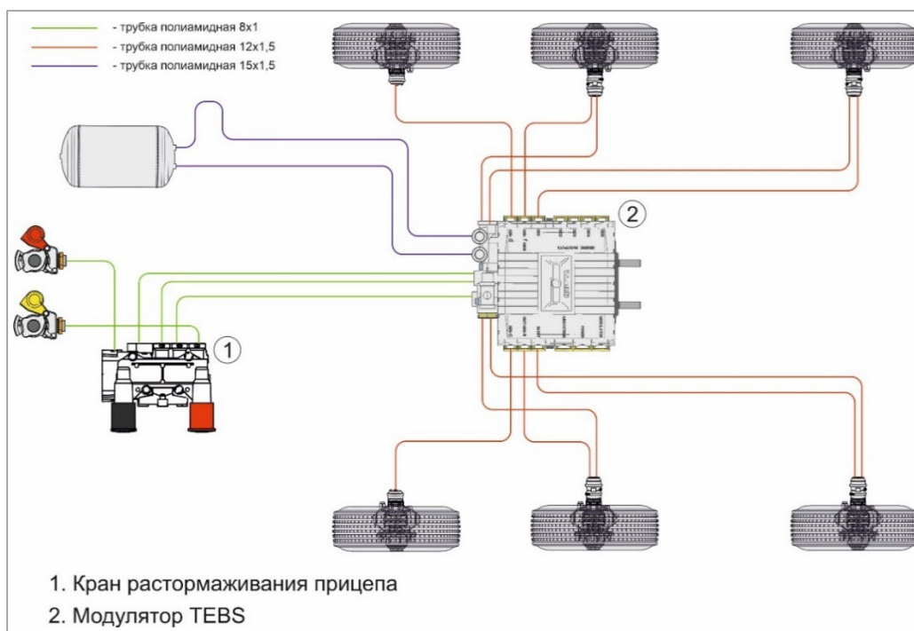
Рис. 29.1. Тормозной контур
