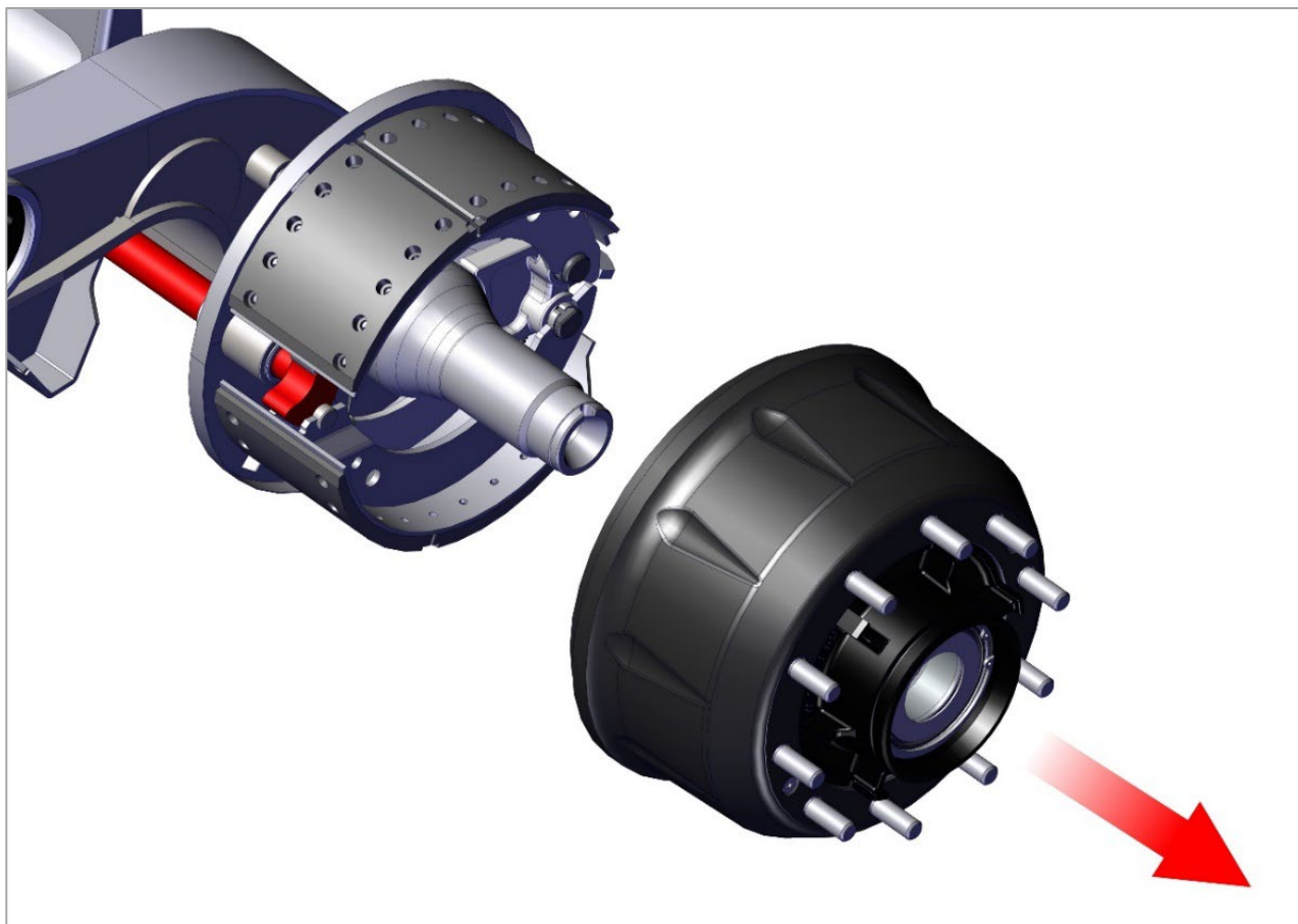
Рис. 16. Снятие сборочного узла ступицы и барабана
