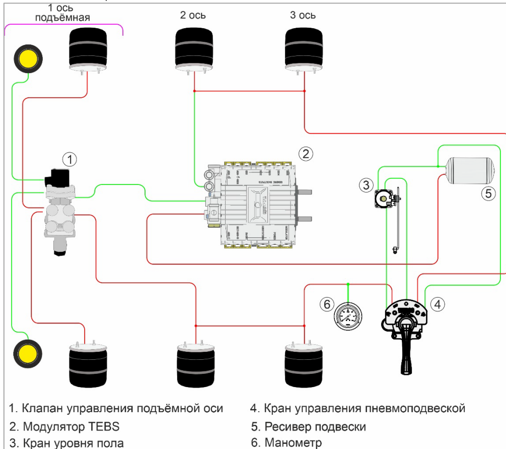
Рис. 29. Контур пневмоподвески
