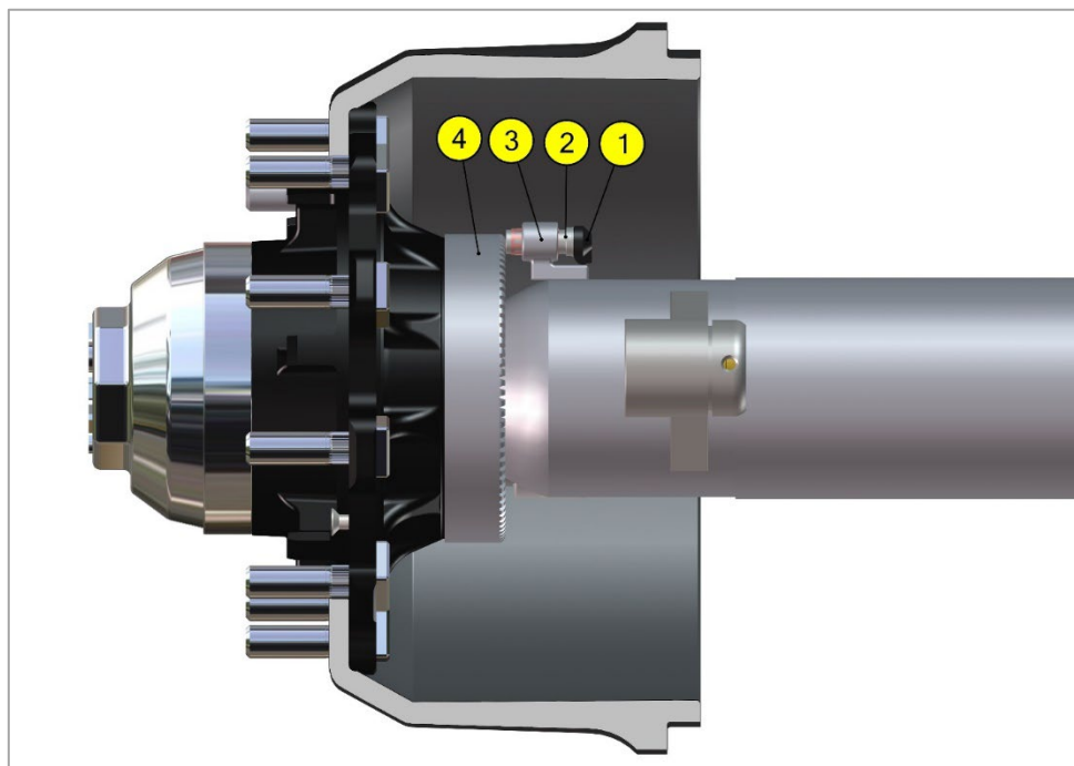
Рис. 11. Датчики ABS
