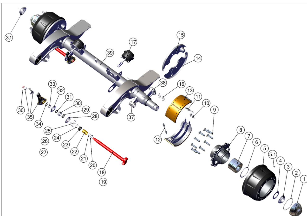
Рис. 10. Взрыв-схема оси полуприцепа с барабанными тормозами
