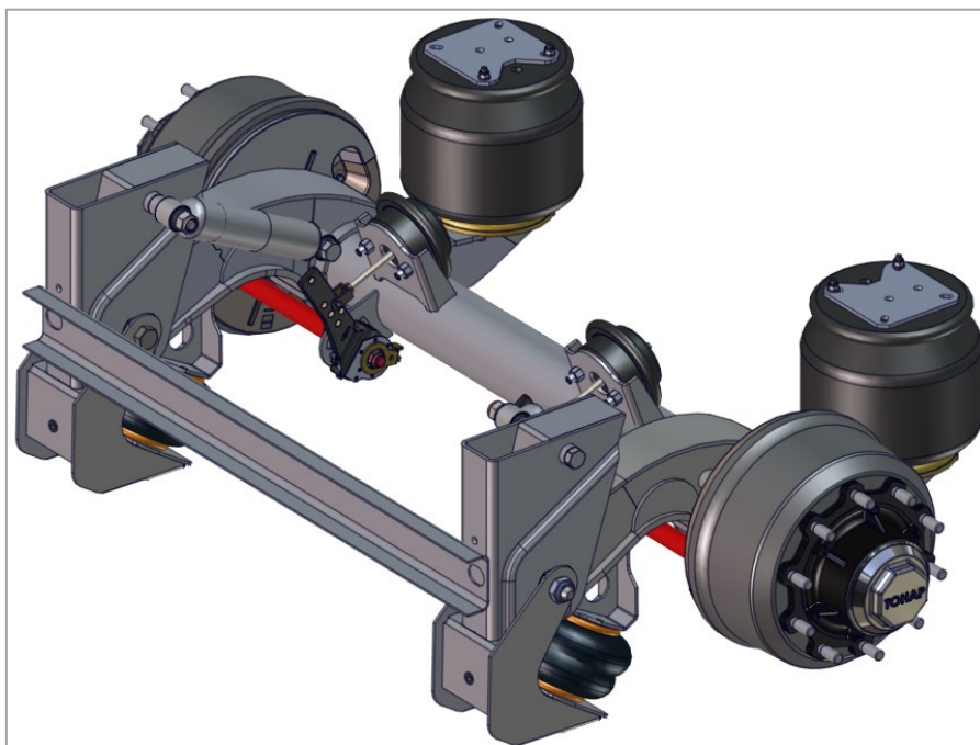
Рис. 5. Рычажная подвеска с барабанными тормозами
