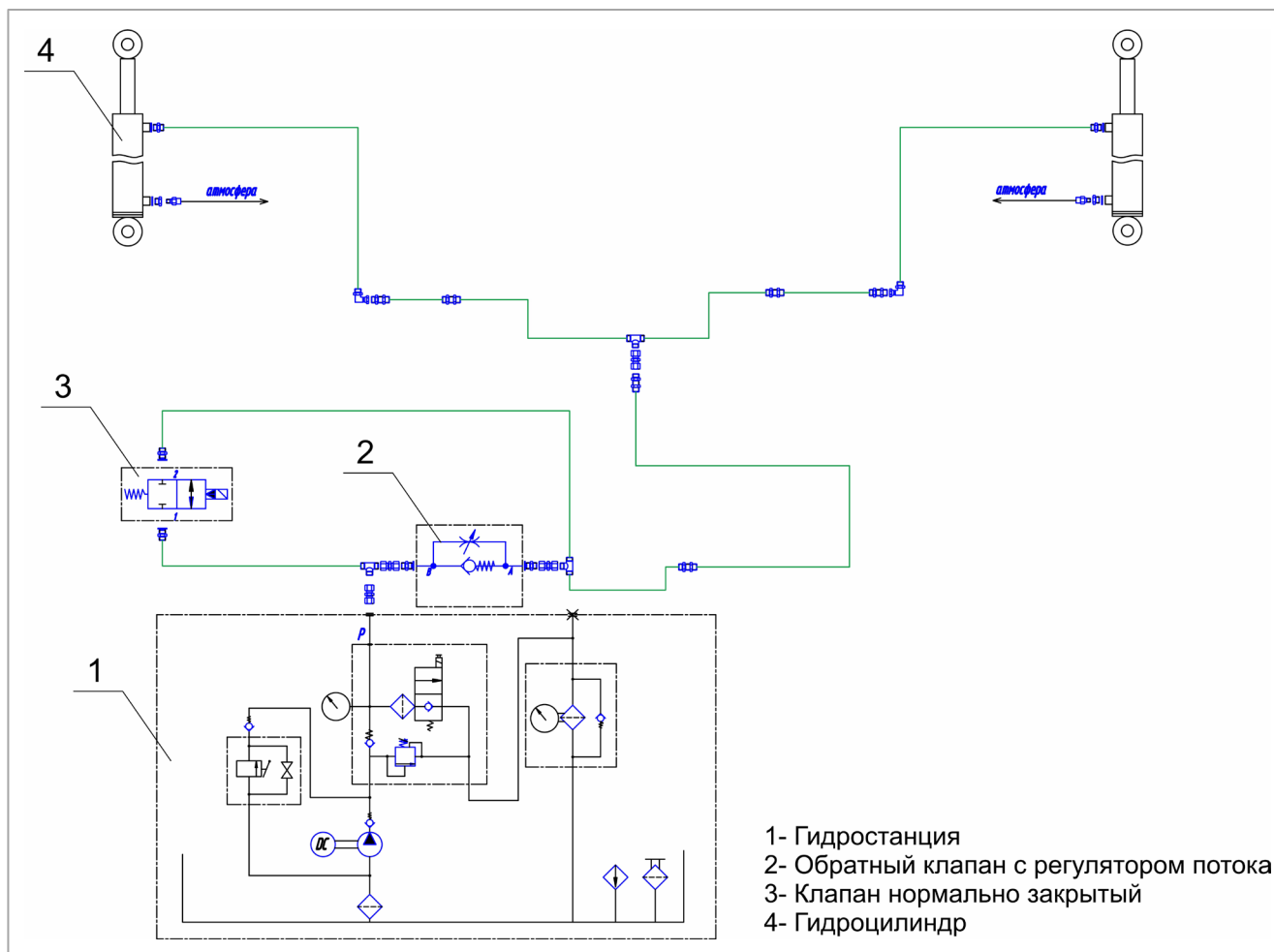
Рис. 33. Гидравлическая схема
