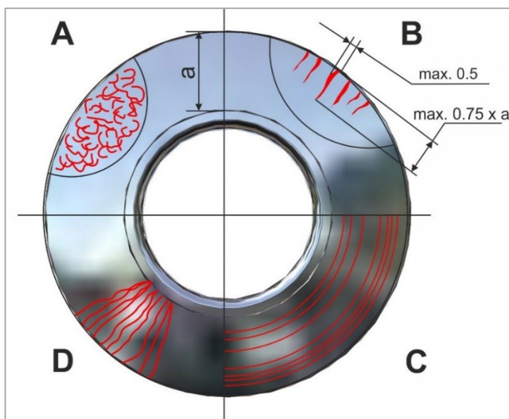
Рис. 26. Состояние рабочих поверхностей
