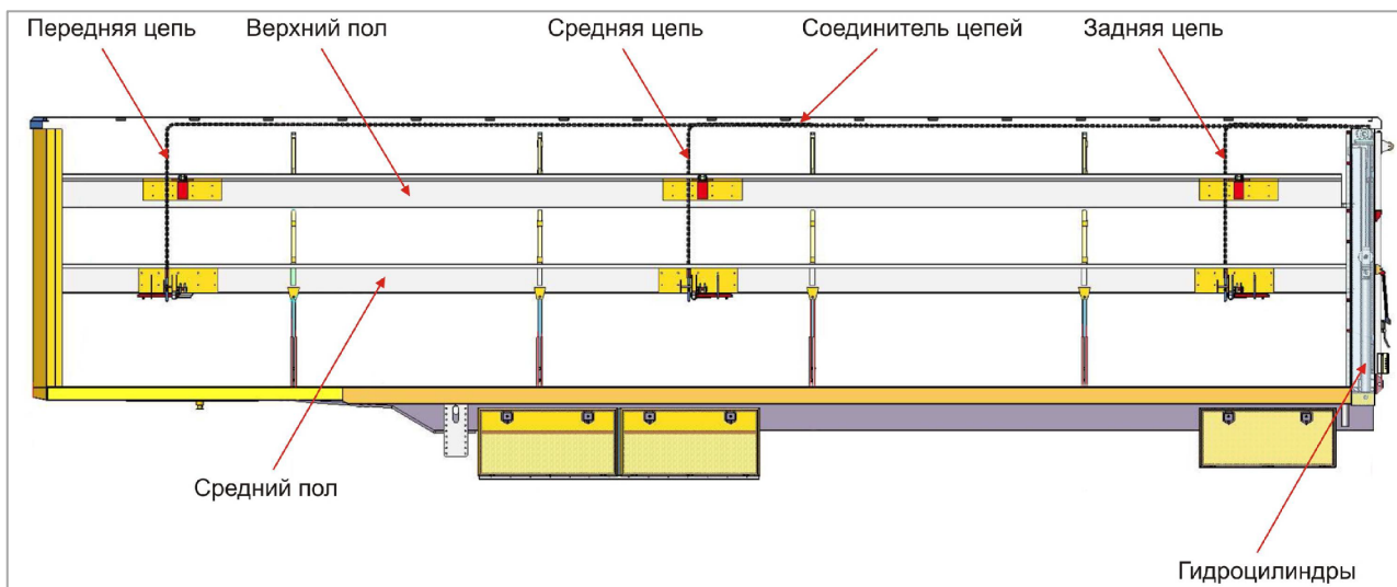
Рис. 35. Схема подъёмных полов
