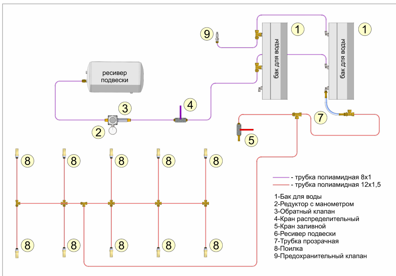
Рис. 38.1 Схема системы подачи воды
