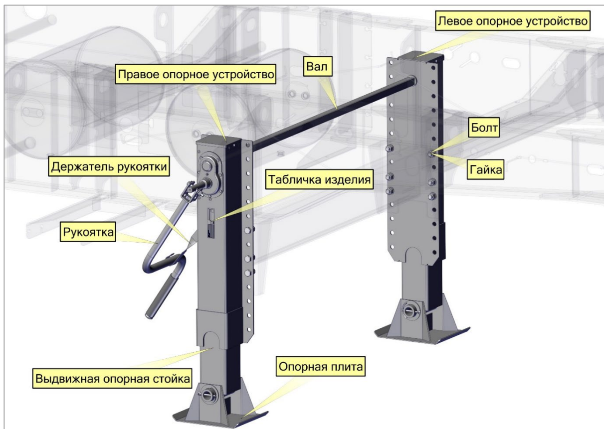
Рис. 31. Опорное устройство
