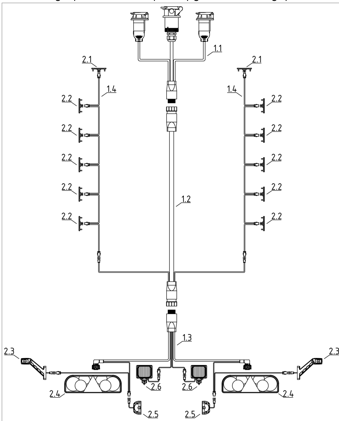
Рис. 32. Электрическая схема
