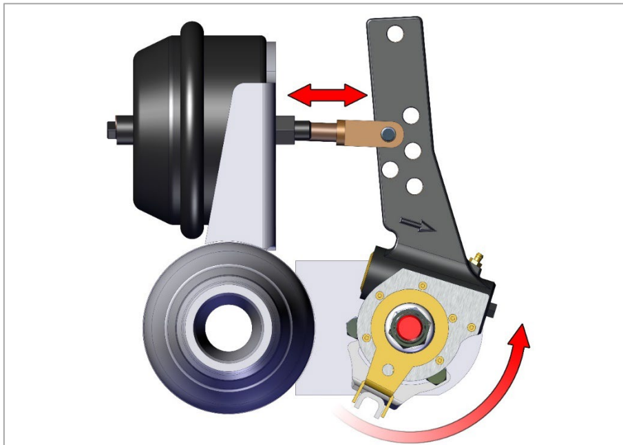
Рис. 21.4. Закрепить регулятор.
