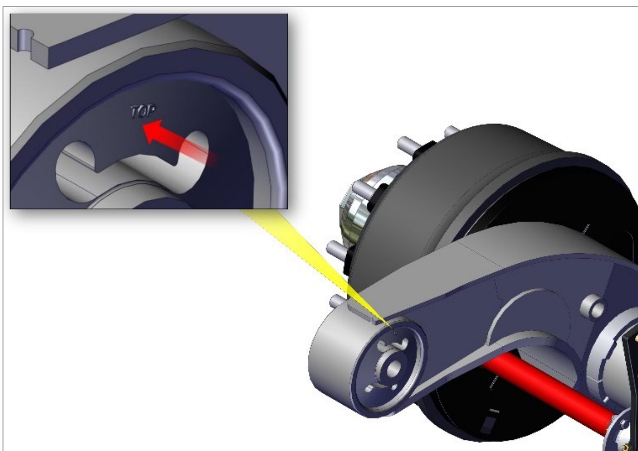
Рис. 9. Установка сайлентблока
