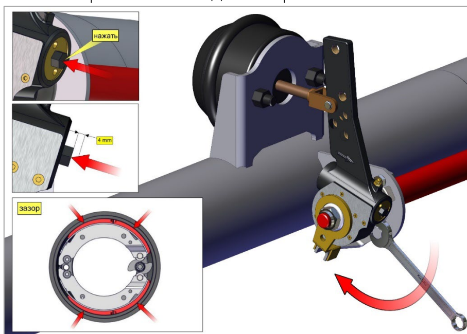
Рис. 21.7. Фиксатор.
