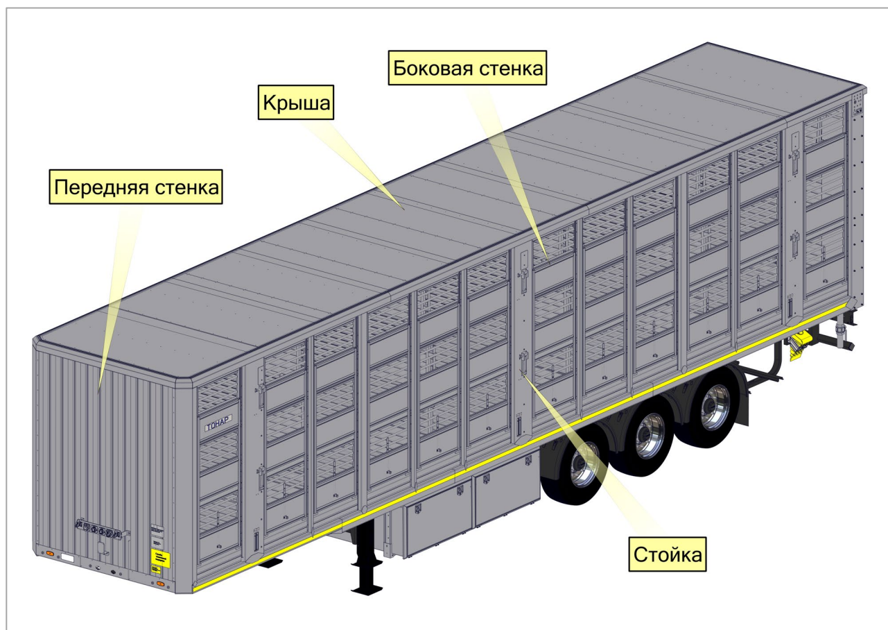
Рис. 3. Кузов полуприцепа
