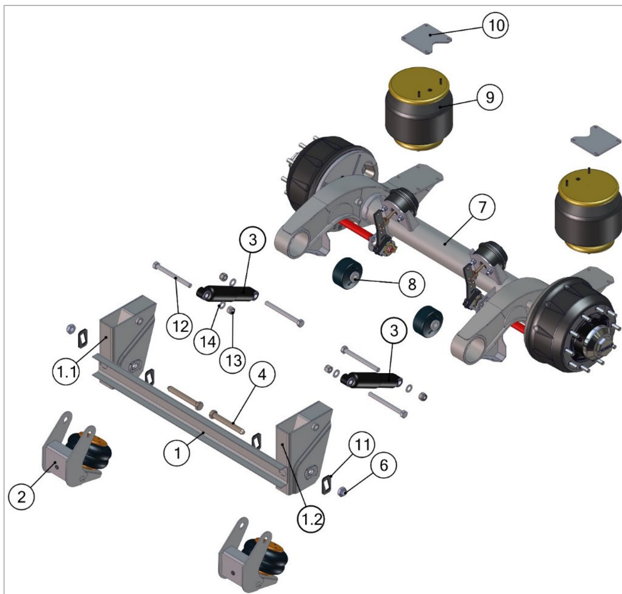
Рис. 7. Взрыв-схема рычажной подвески с барабанными тормозами
