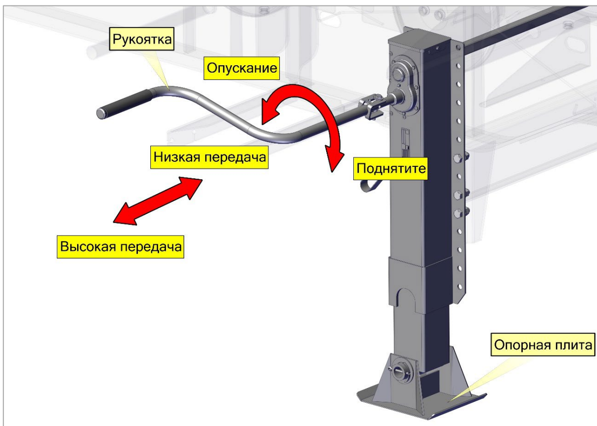
Рис.7 Управление опорным устройством
