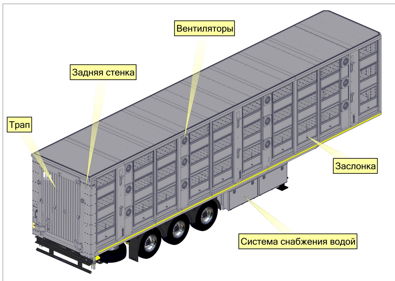
Рис. 4. Кузов полуприцепа
