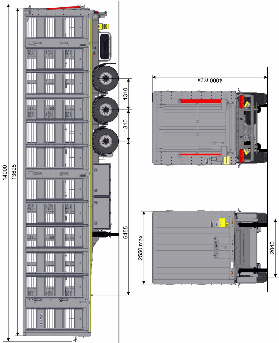
Рис.40. Габаритный чертёж модели 9827.
