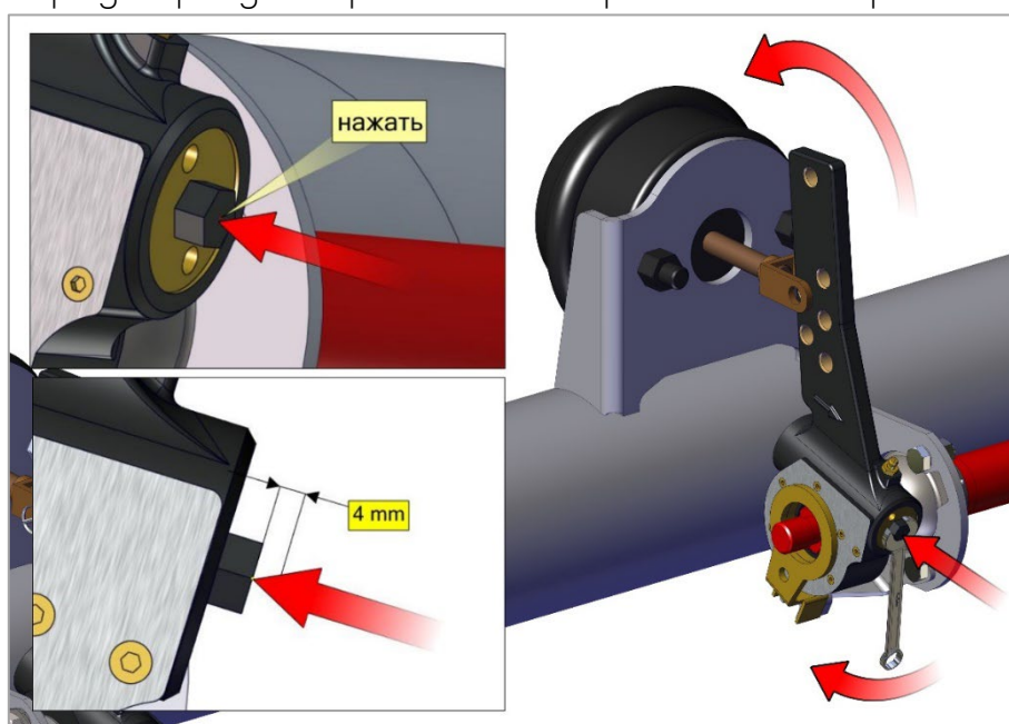
Рис. 21.1. Фиксатор.
