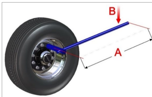
Рис. 28. Затяжка гаек
