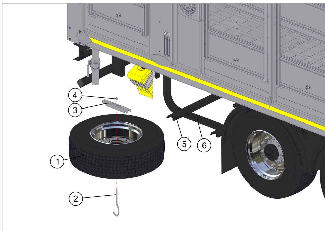
Рис. 39. Установка запасного колеса
