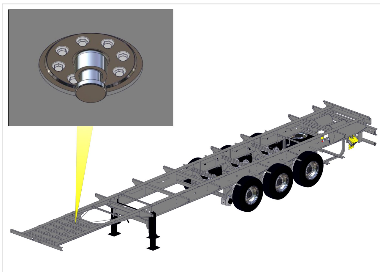
Рис. 1. Рама полуприцепа
