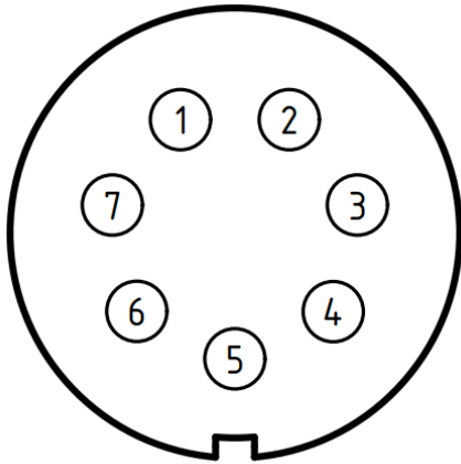
вид на розетку полуприцепа
