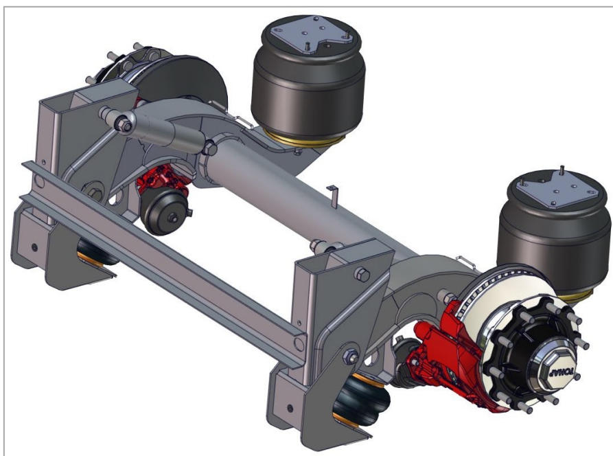
Рис. 6. Рычажная подвеска с дисковыми тормозами
