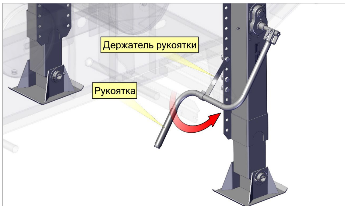
Рис.6 Достать рукоятку
