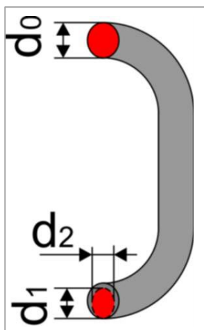
Рис. 34.1. Уменьшение диаметра сечения звена
