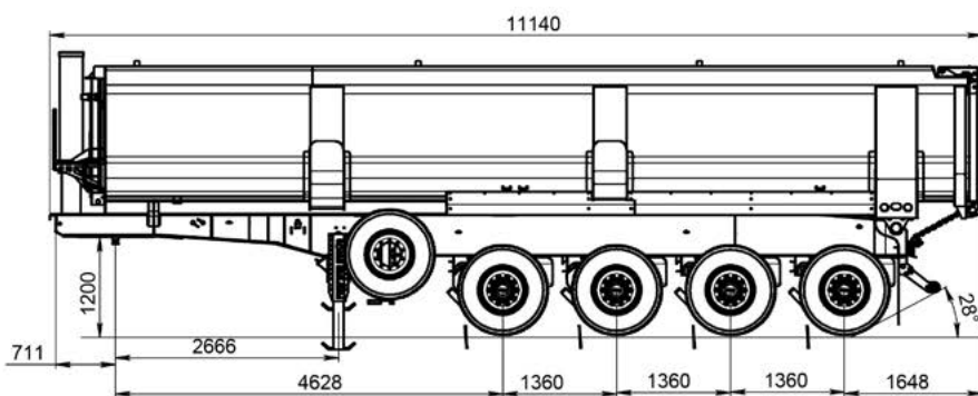
Габаритный чертеж модели 95234
