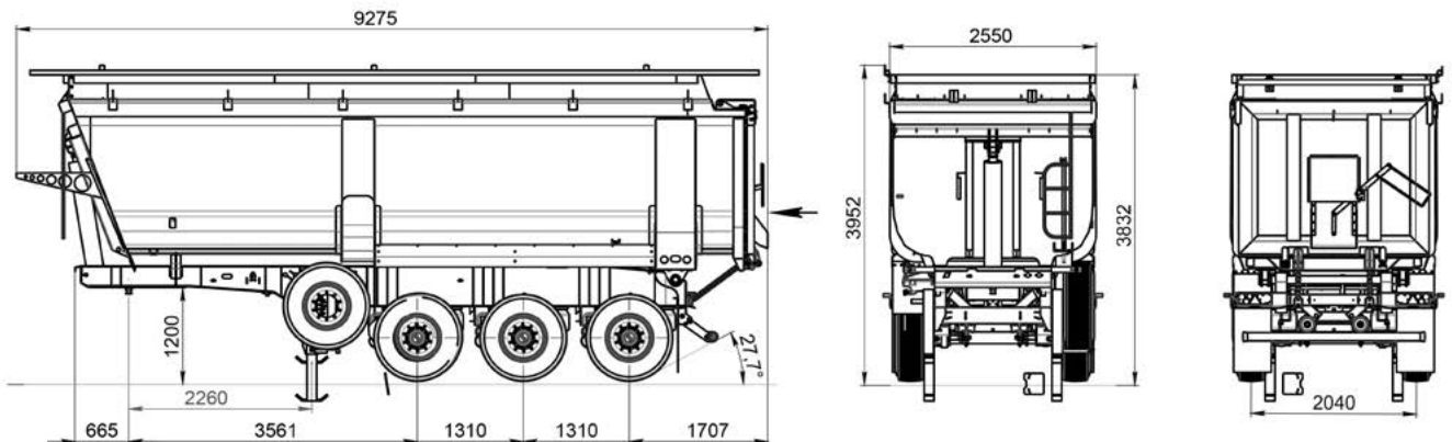
Габаритный чертеж модели V=30 куб.м
