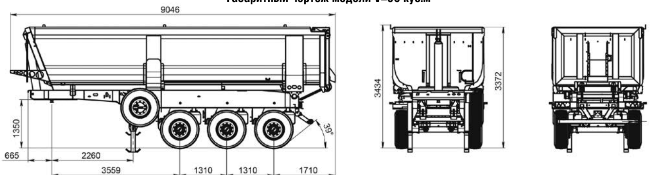
Габаритный чертеж модели V=30 куб.м
