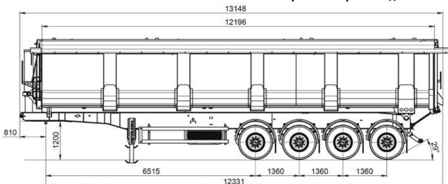
Габаритный чертеж модели 952342
