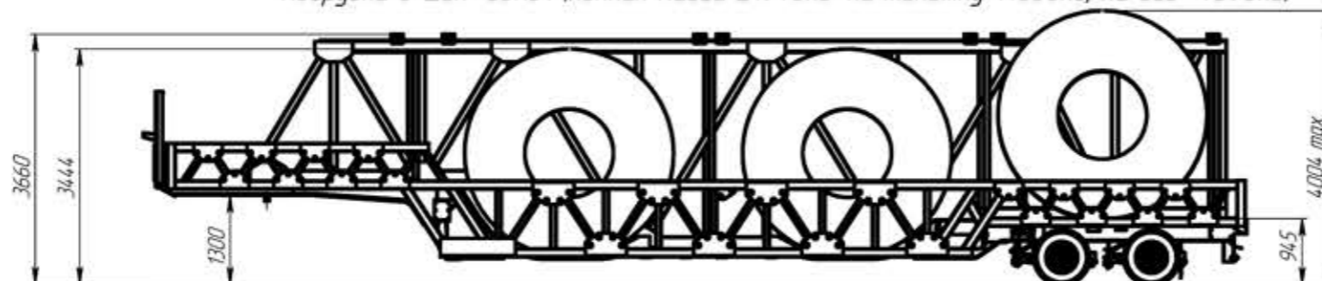
Погрузка 6 шин 33R51 (полная масса 21940кг: на тележку 14350кг, на ССУ 7590кг)
